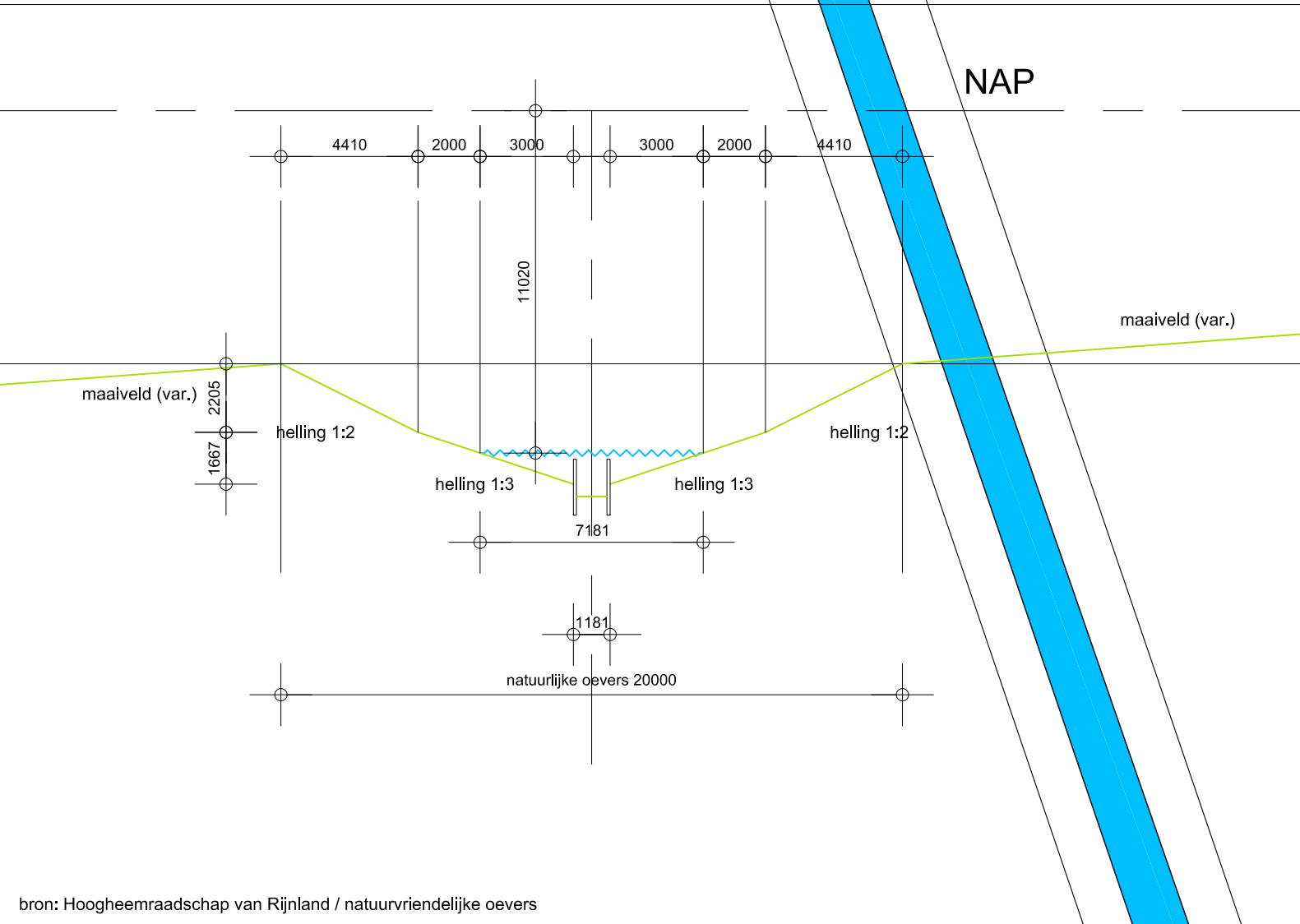
doorsnede A natuurvriendelijke oevers
