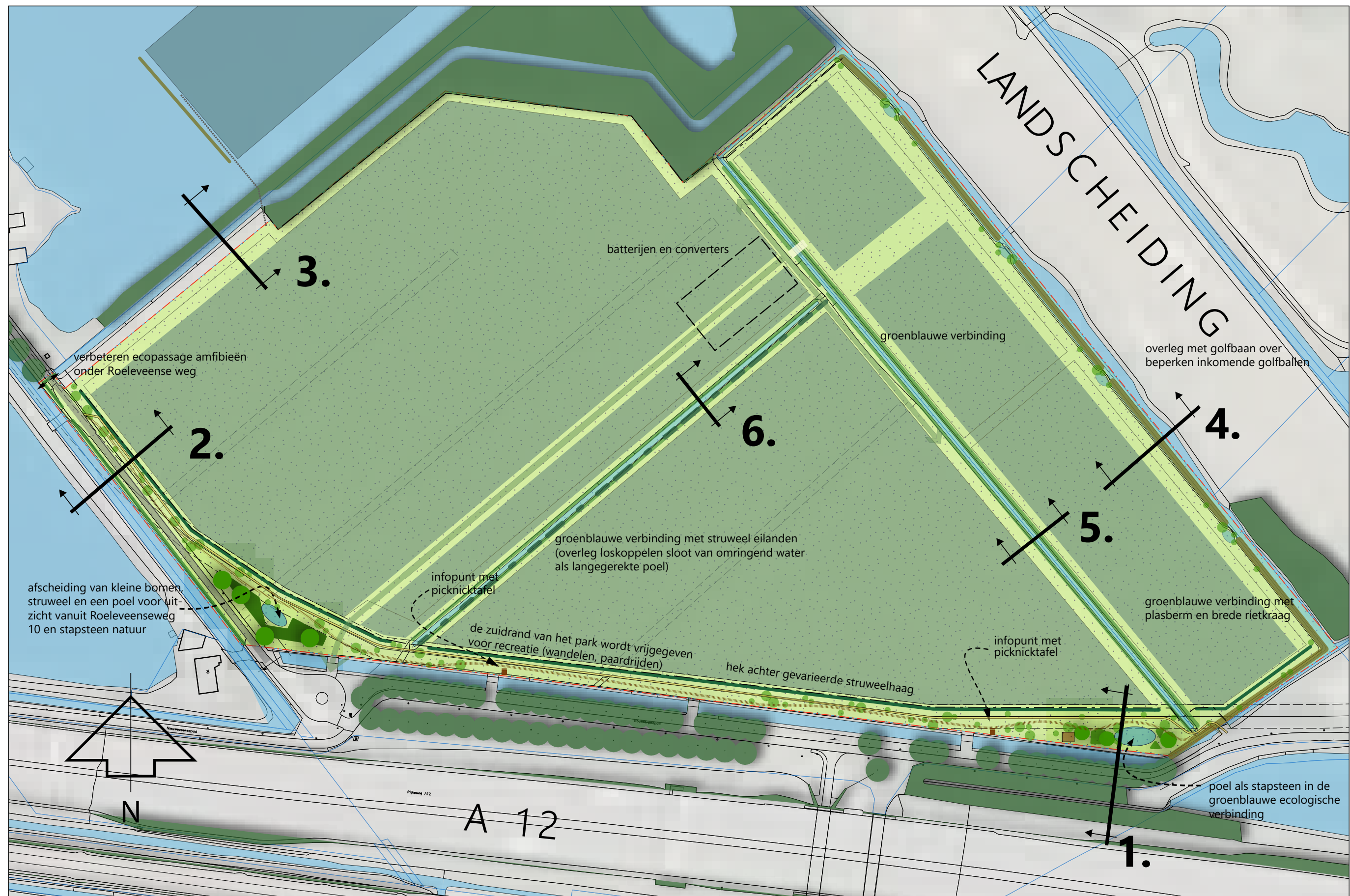
afb. 16: structuurschets (www.haverdroeze.nl)
