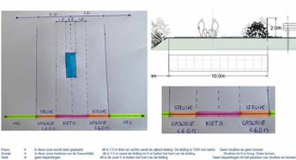
afb. 42: beperkingen vrijwaringszone en vergelijking met profiel 1 (leidingbeheerder)
