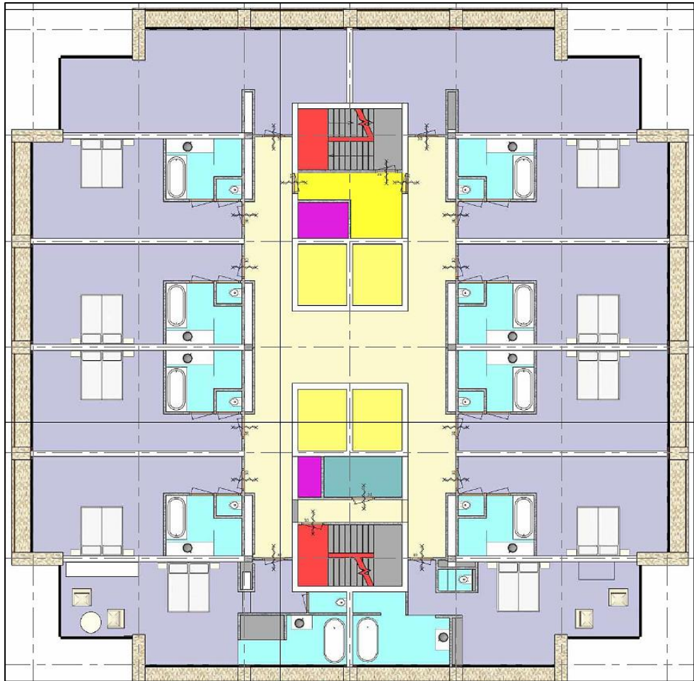
Impressie verdiepingen (bron: P.A.M. Teunissen Architectenburo)
