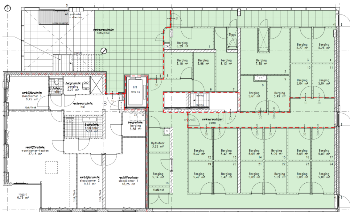
Afbeelding 1: Begane grond
