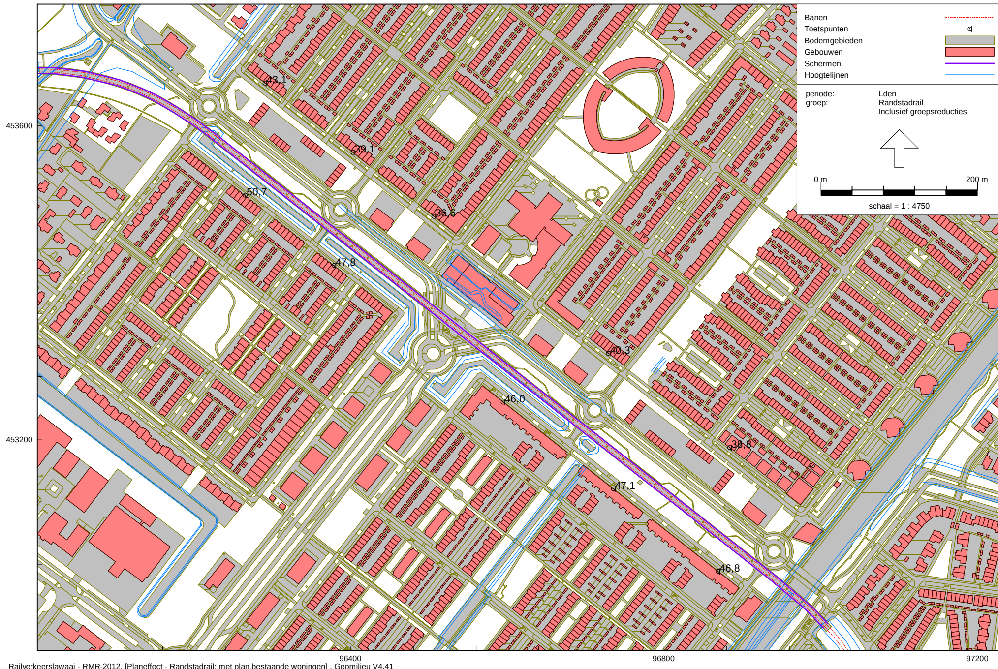
Geluidsbelasting railverkeer bestaande woningen Situatie met bebouwing plan
