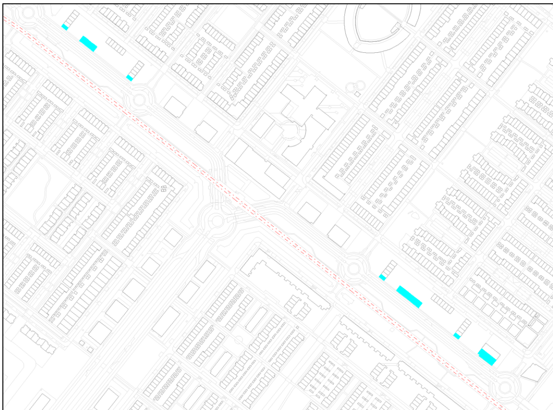
Afbeelding 8 : Hogere waarden Randstadrail (lichtblauw tot en met 50 dB)
