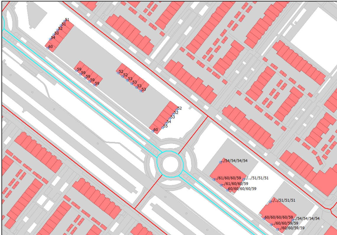
Afbeelding 7 : Hogere waarden Hugo de Grootlaan
