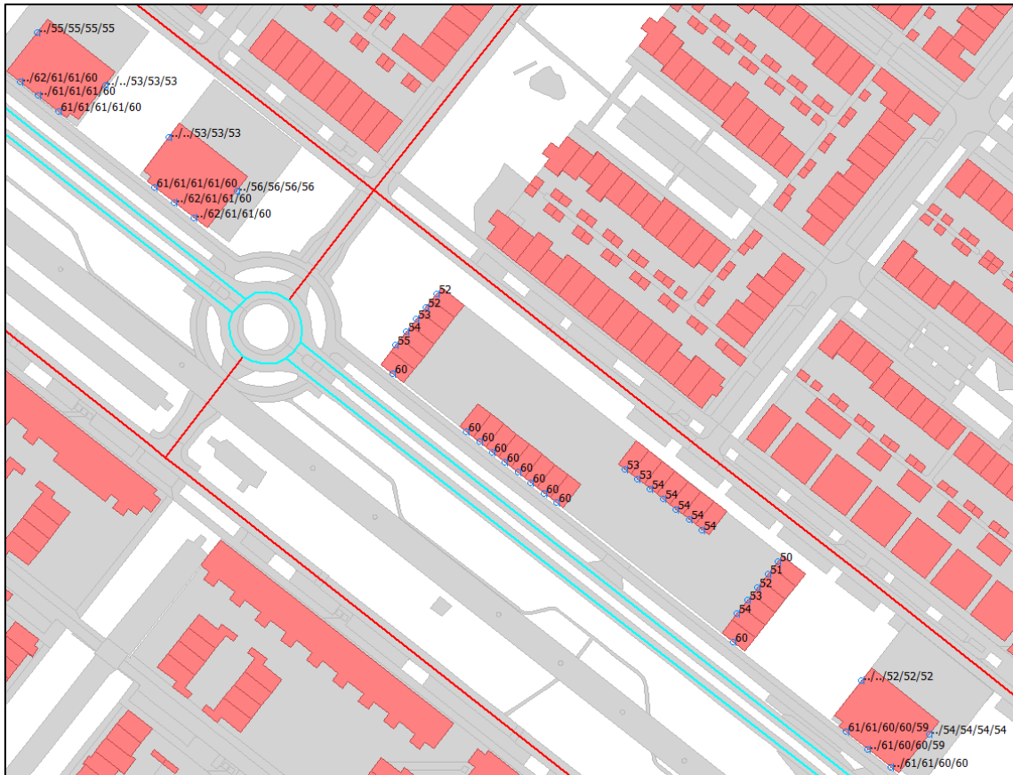
Afbeelding 6 : Hogere waarden Aletta Jacobslaan
