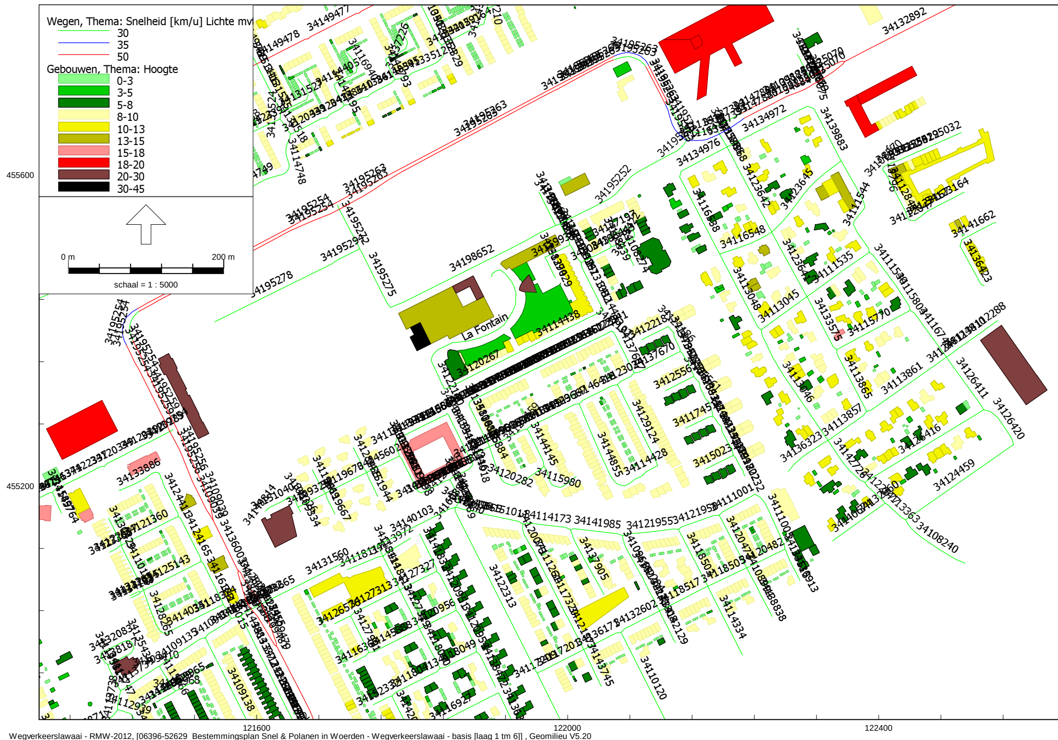
Figuur II-4 Overzicht wegen, rijnsnelheden en gebouwhoogten
