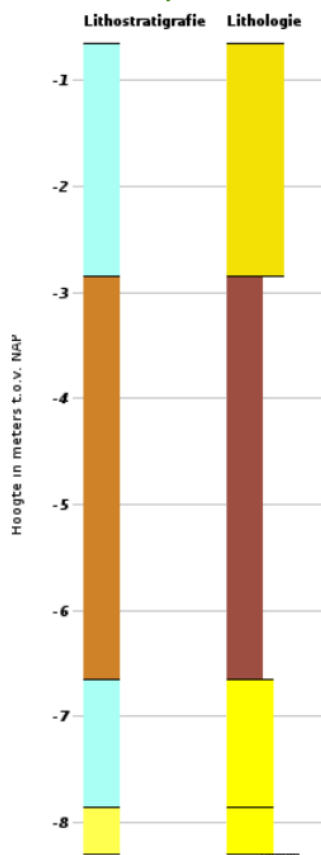
Figuur 23: Geologisch boorprofiel B31G2033 (Dinoloket 2014).
