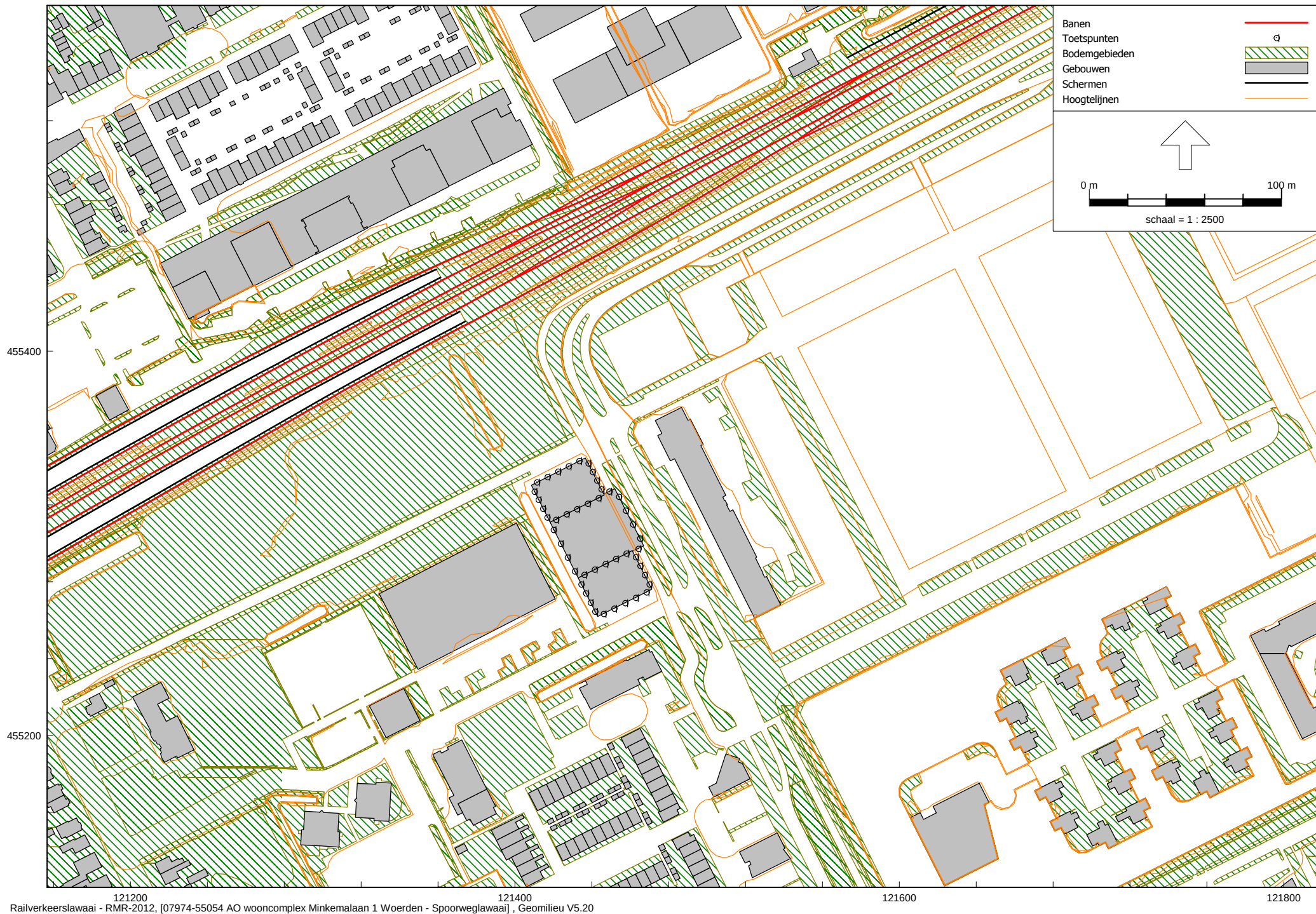
Figuur II-1 Overzicht rekenmodel spoorweglawai
