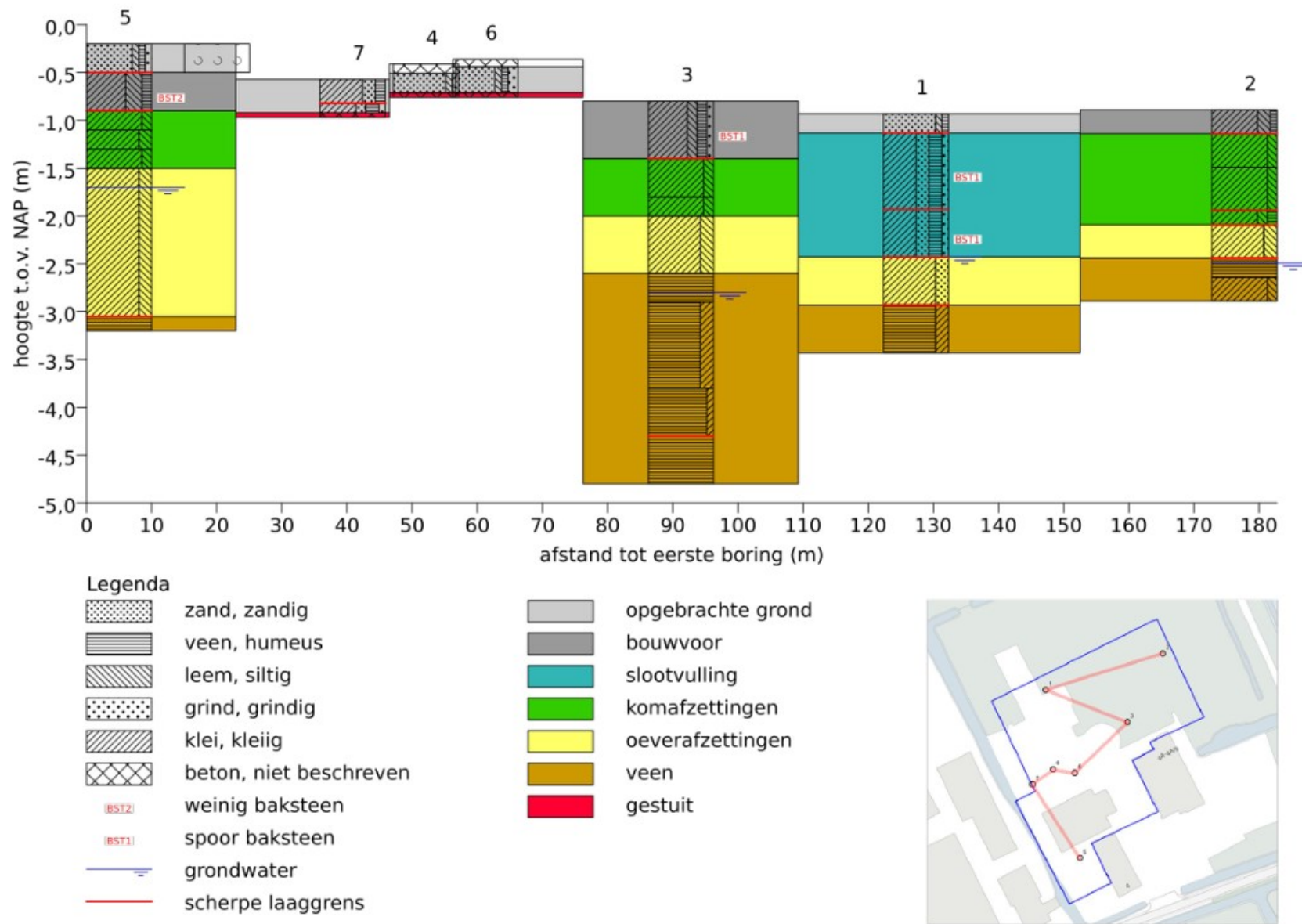
Figuur 31: Schematische zuid-noord doorsnede van de boorprofielen.
