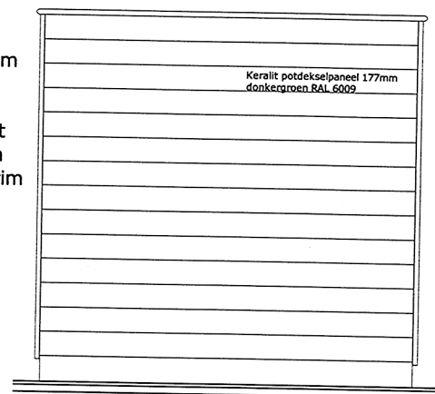
Aanzicht ZO zijde
