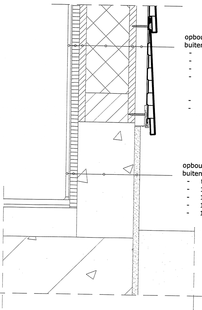
Vertikaal detail 2: aansluiting gevel-vloer-maaiveld
