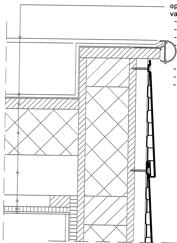
Vertikaal detail 1: aansluiting gevel-dak
