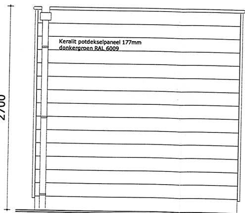
Aanzicht NW zijde
