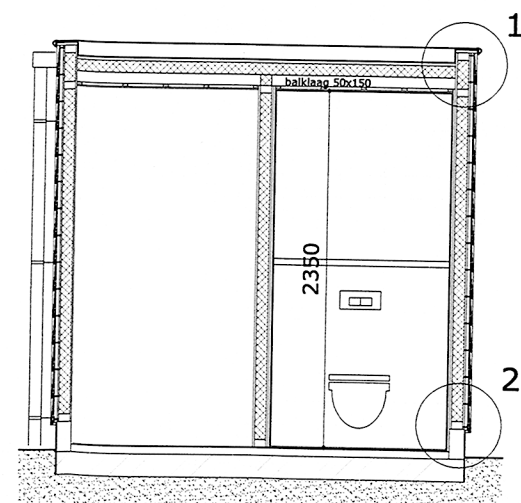
Dwarsdoorsnede
