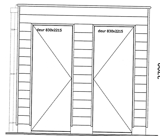
Aanzicht ZW zijde
