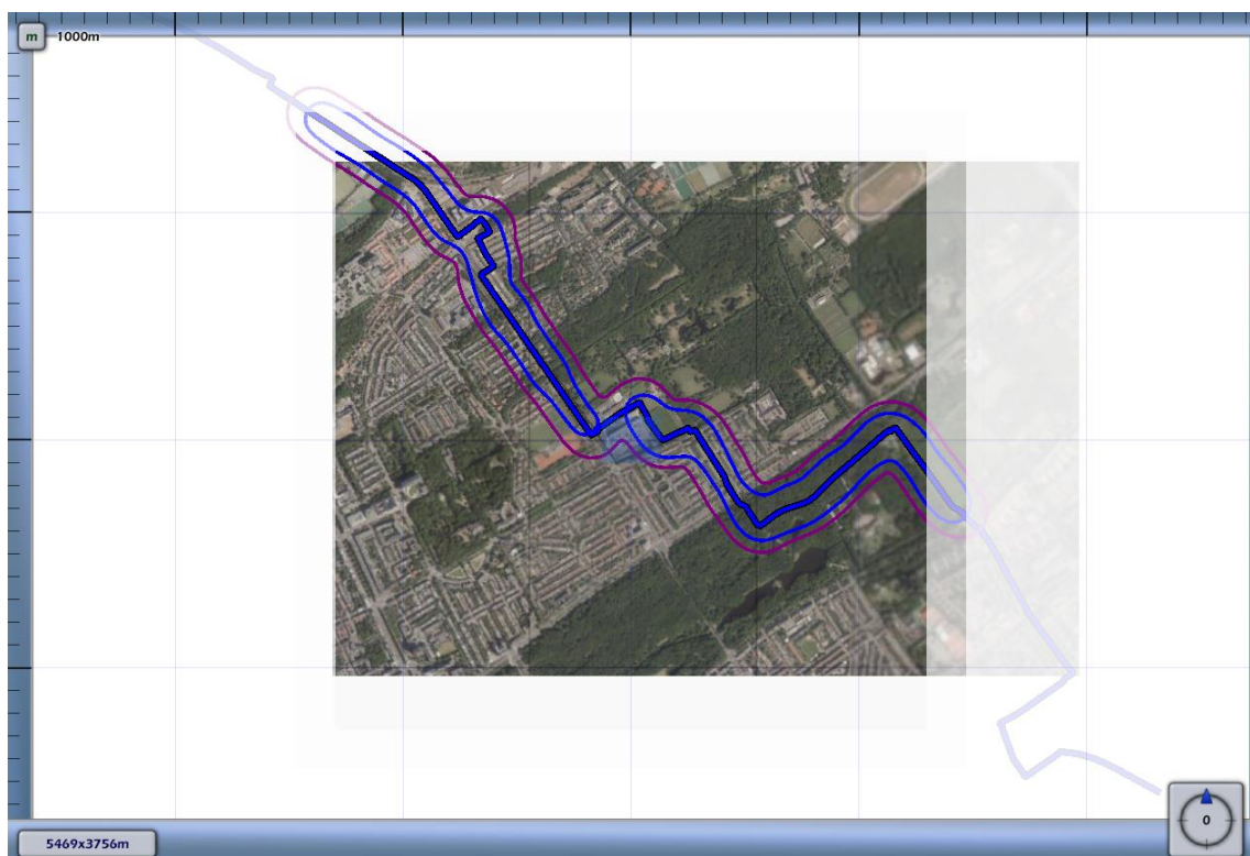
3.1 Figuur 3.1 Plaatsgebonden risico voor 7945_leiding-W-514-16-deel-1 van N.V. Nederlandse Gasunie
