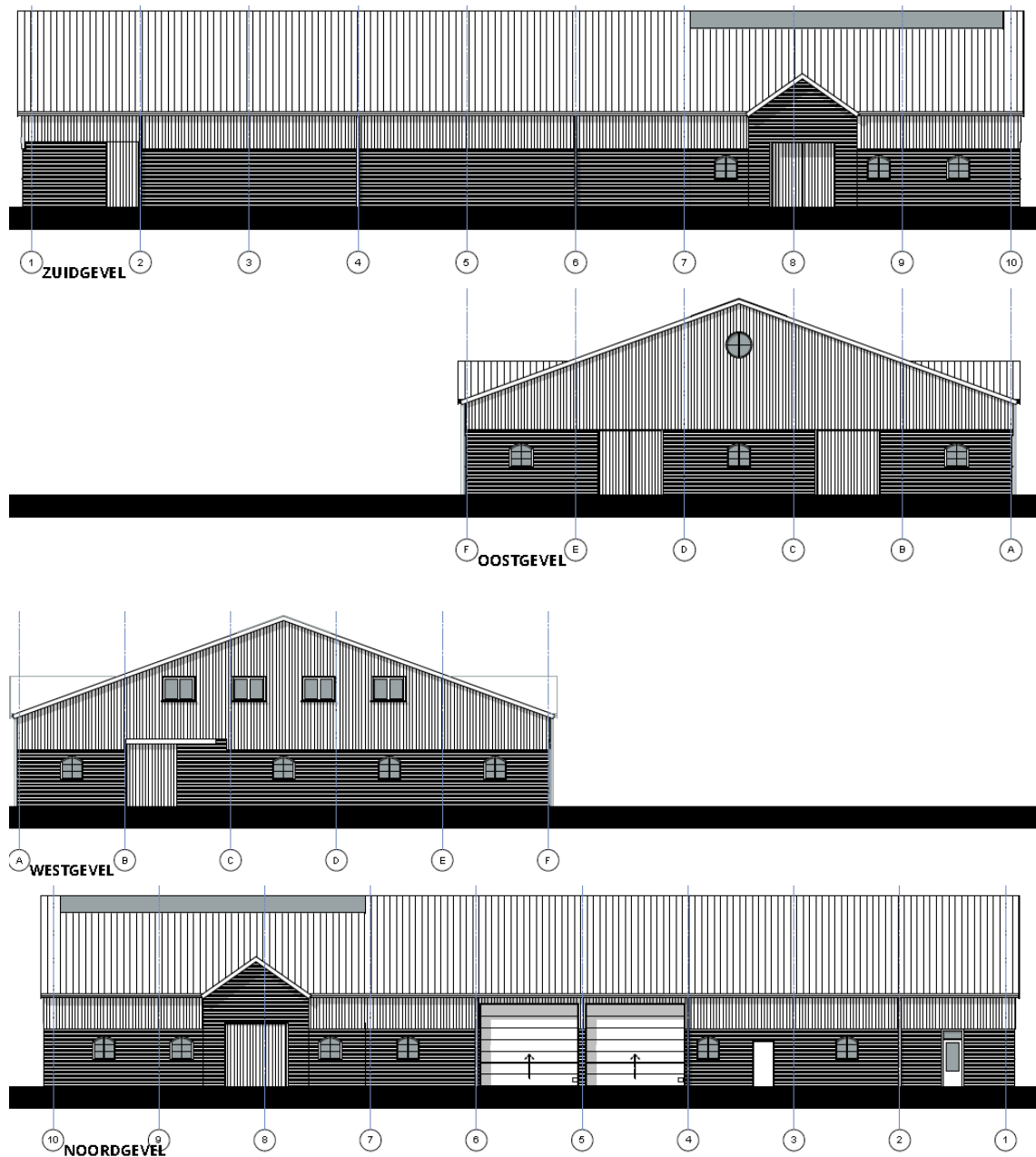
Figuur 4: Aanzichttekeningen stal.
