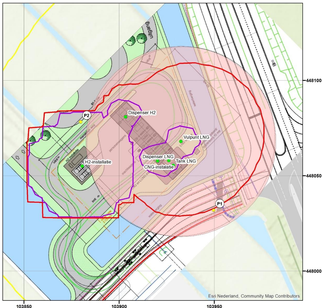
Figuur 5. Ministerie I&M interim beleid LNG-tankstations (roze gebied rond het vulpunt met een straal van 50 m) en de grenswaarde van het plaatsgebonden risico (rode contour)
