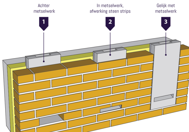
Figuur 122: Mogelijkheden plaatsing van vleermuiskasten in een gevel
