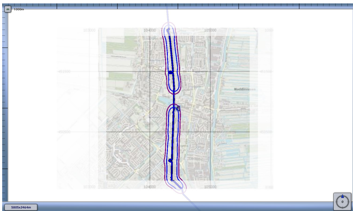
3.1 Figuur 3.1 Plaatsgebonden risico voor 7424_leiding-W-517-01-deel-1 van N.V. Nederlandse Gasunie
