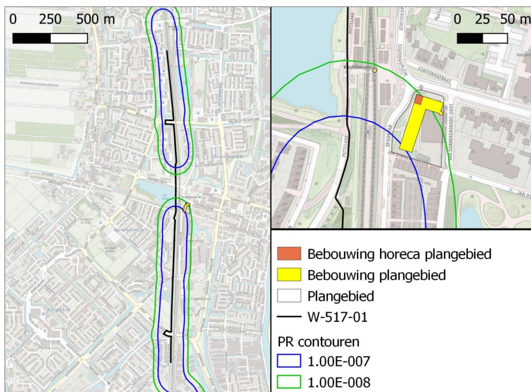
Figuur 2. Plaatsgebonden risicocontouren aardgasbuisleiding W-517-01
