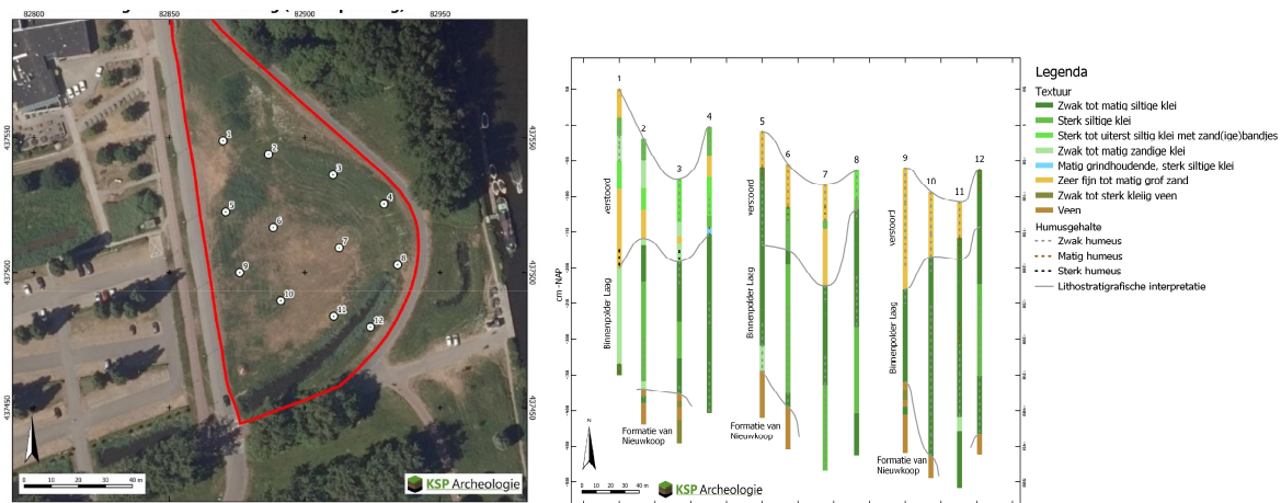
Afbeelding 3: Boorpunten en profielen KSP Archeologie 2022 3
