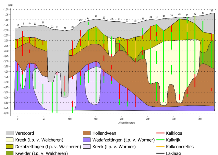
Figuur 10. Profiel over de westelijke helft van deelgebied Watersportweg.
