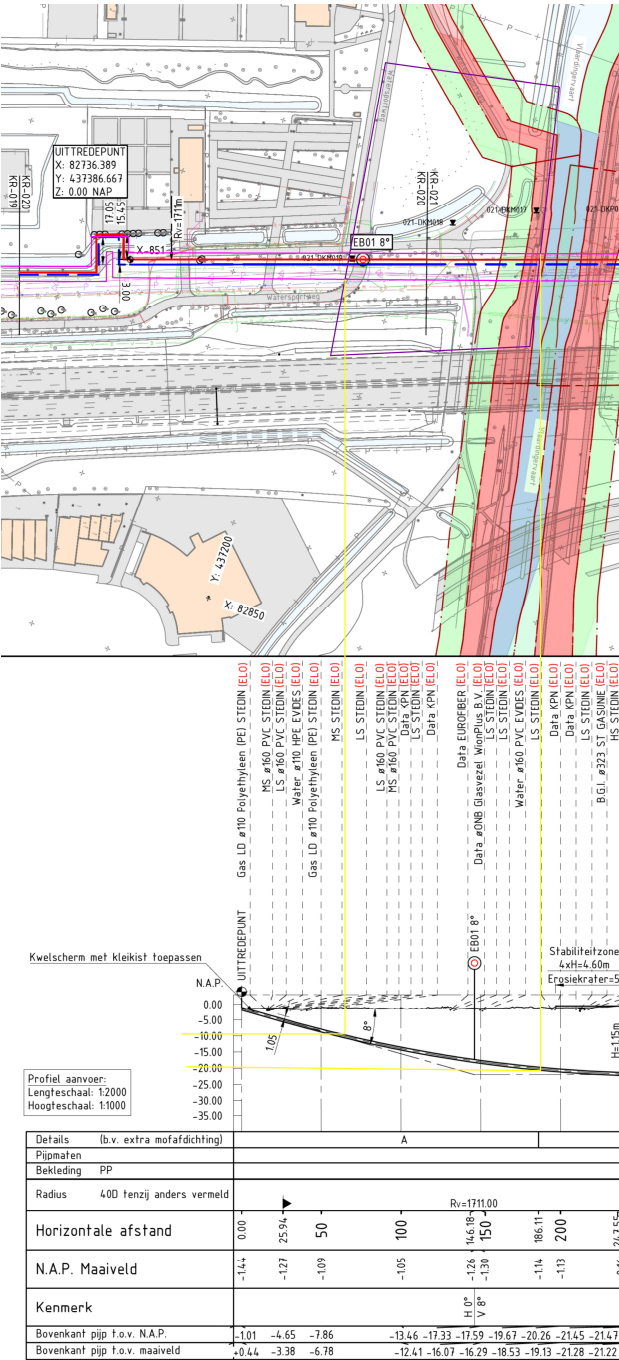
Afbeelding 1: Warmtetransportleiding, tracé en diepte met aanduiding ligging AMK terrein 16131
