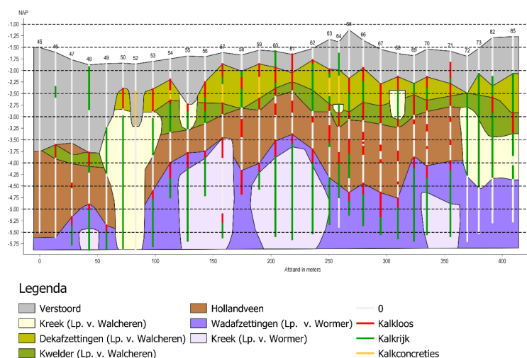
Afbeelding 3, boorprofielen RAAP ten noorden van de A20 2
