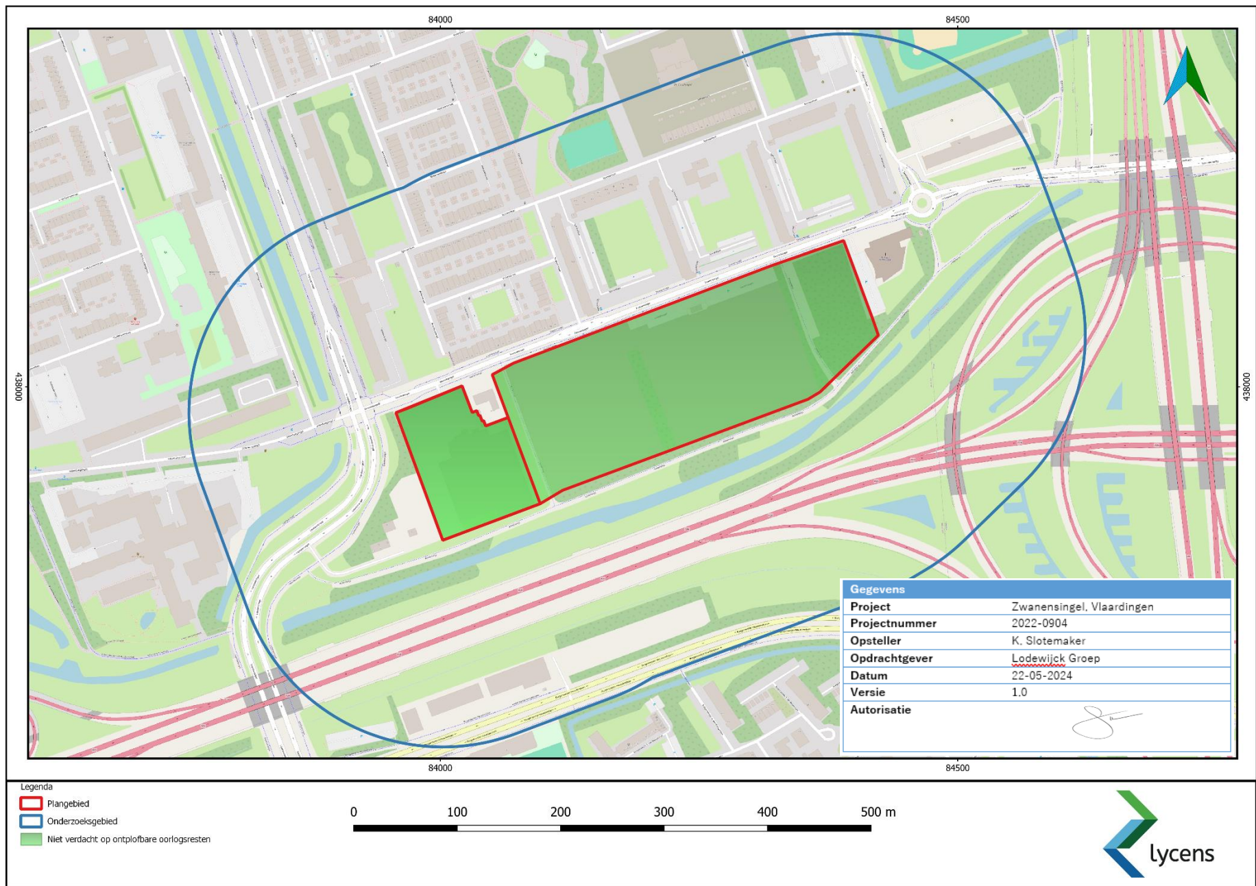
Afb. 14 Bodembelastingkaart na-conflict
