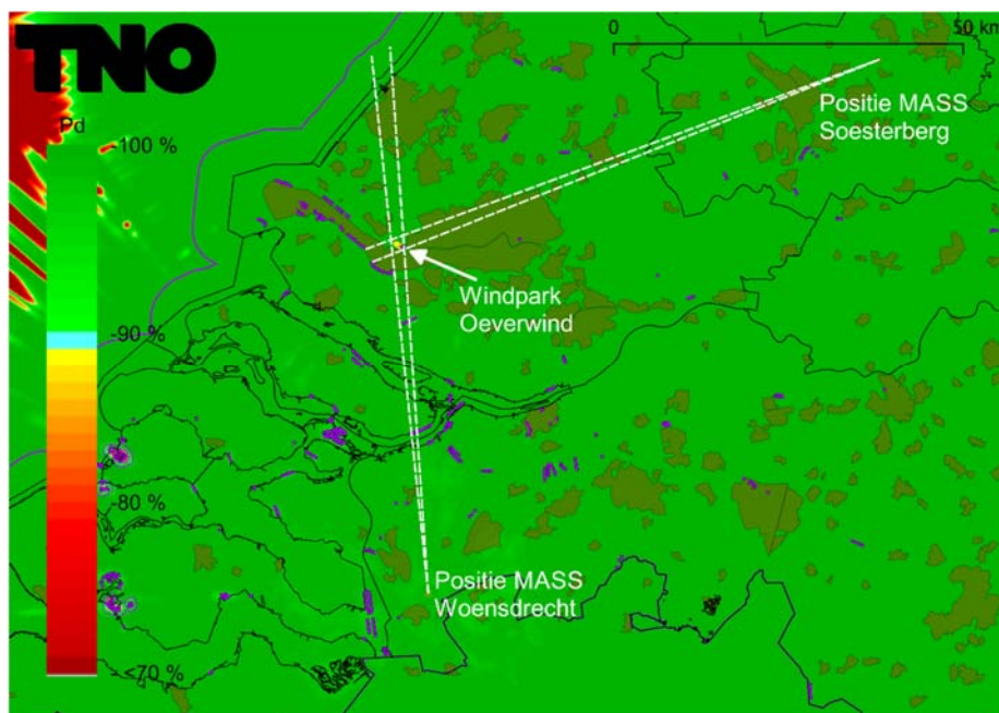
Figuur 9 Detectiekans van het primaire verkeersleidingsradarnetwerk berekend op 1000 voet in het schaduwgebied van bouwplan nadat deze is gerealiseerd. Op dit figuur is detectiekansmiddeling toegepast. De stippellijnen geven aan waar de schaduw kan ontstaan.
