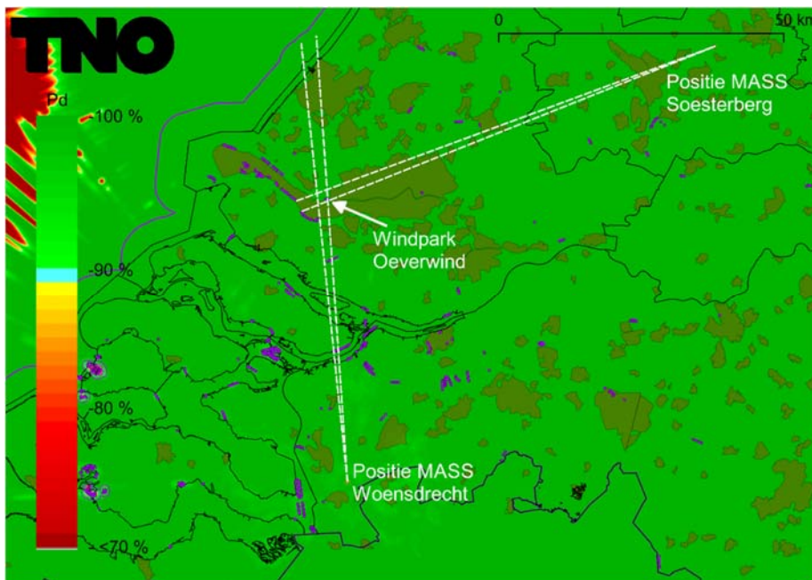
Figuur 8 Detectiekans van het primaire verkeersleidingsradarnetwerk op 1000 voet in het schaduwgebied van bouwplan voordat deze is gerealiseerd (baseline). Op dit figuur is detectiekansmiddeling toegepast. De stippellijnen geven aan waar de schaduw kan gaan ontstaan.
