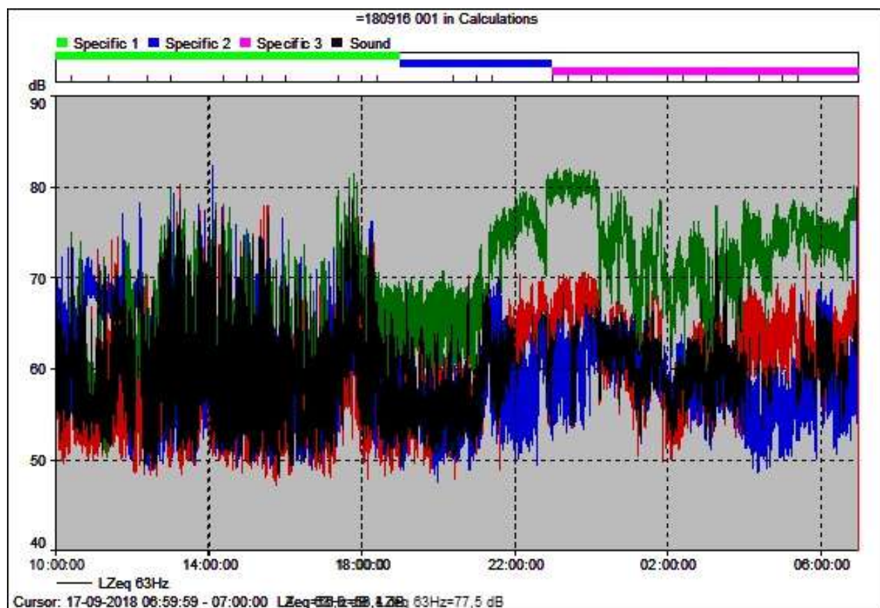
Figuur 6.3: Vergelijking verloop geluidniveau 63 Hz tertsband in de avond en nacht van 16 september. Meetpunt 1 (groene lijn), meetpunt 2 (rode lijn) en meetpunt 3 (blauwe lijn). Zwarte lijn gevolg van samenvallen geluidniveau verschillende meetpunten
