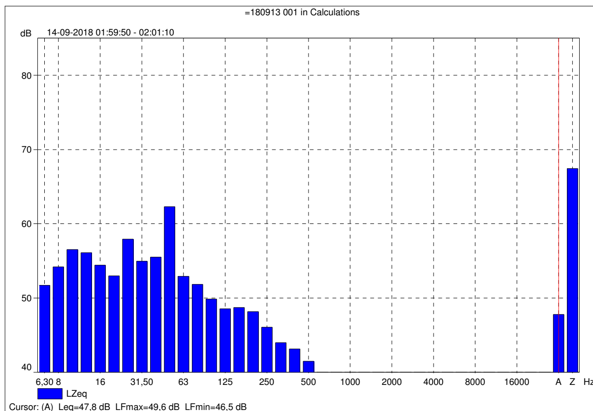
Figuur 7.3: Geluidspectrum meetpunt 2 voor geluidfragment op 14 september om 02.00 uur
