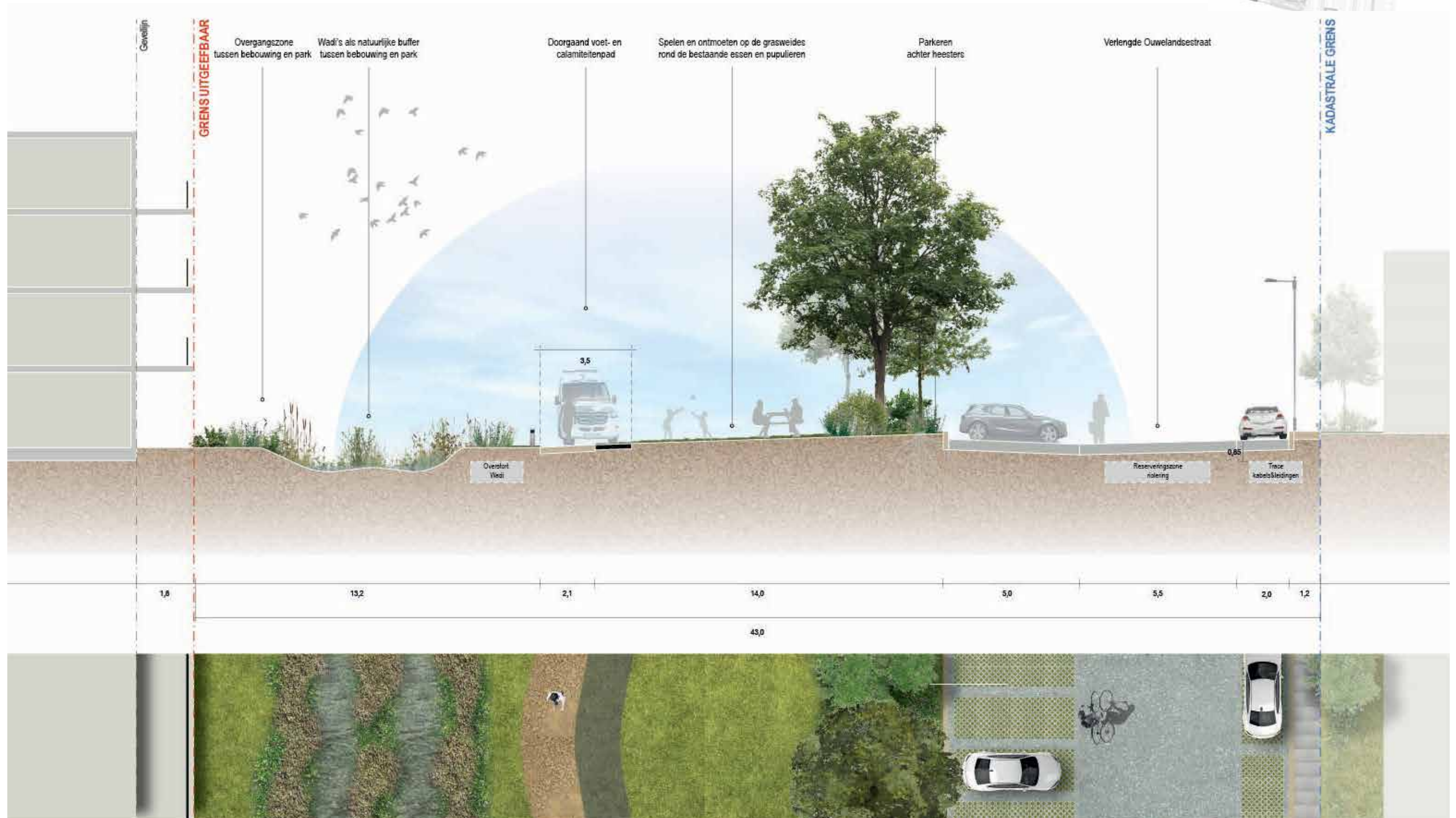
Afbeelding 1 Profiel Oudelandseweg
