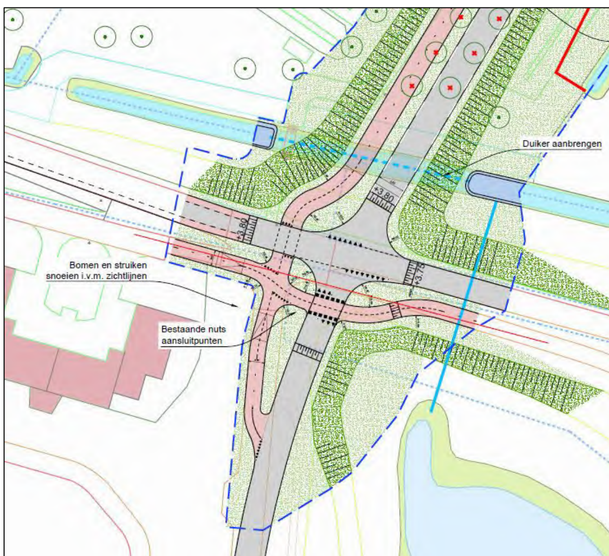
Afbeelding 7: Aan te leggen duiker bij kruising ontsluitingsweg
