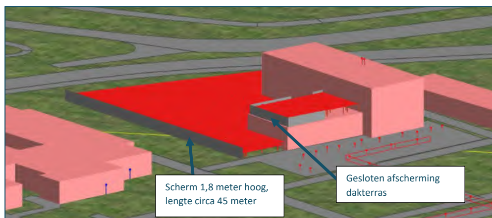
Figuur 8 3D-impressie rekenmodel
