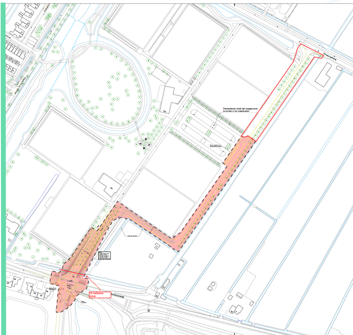
Afbeelding 2: ontwerptekening
