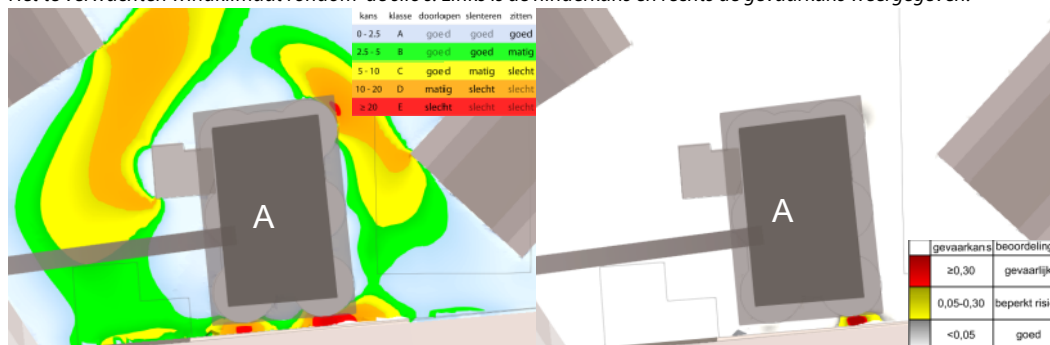
f3.3 Het te verwachten windklimaat rondom de silo's. Links is de hinderkans en rechts de gevaarkans weergegeven.
