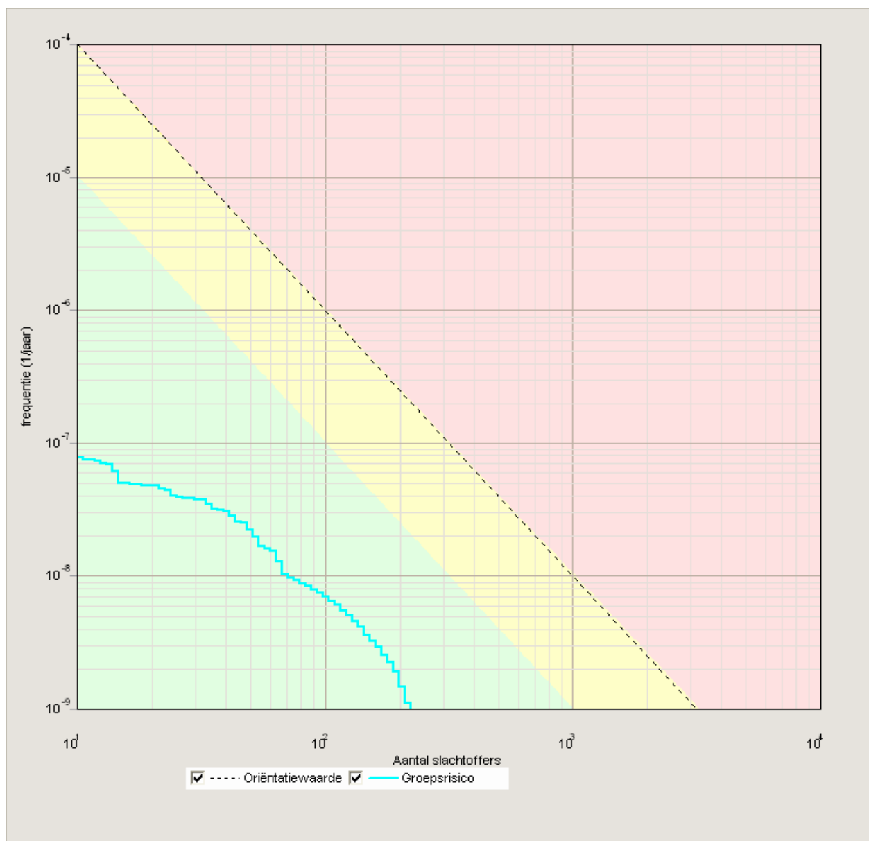
Figuur 4 grafiek groepsrisico A20
