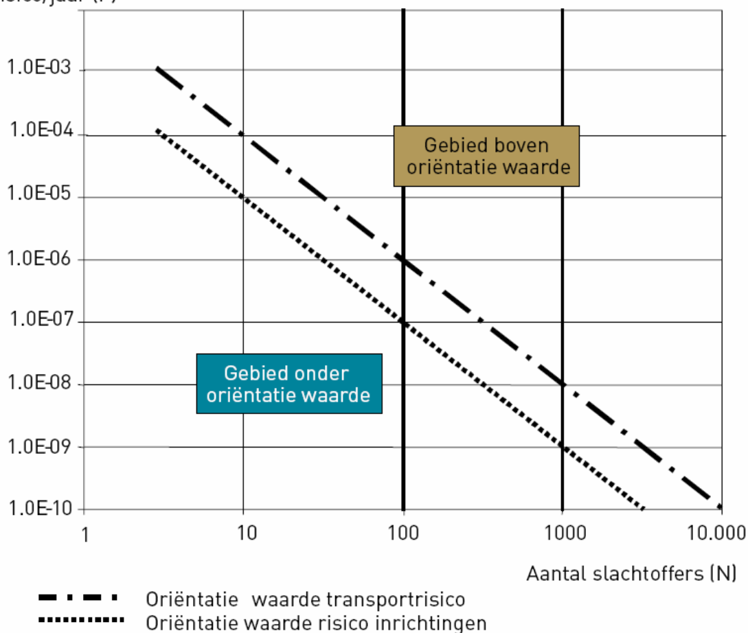
figuur 5: voorbeeld fN-curve groepsrisico
