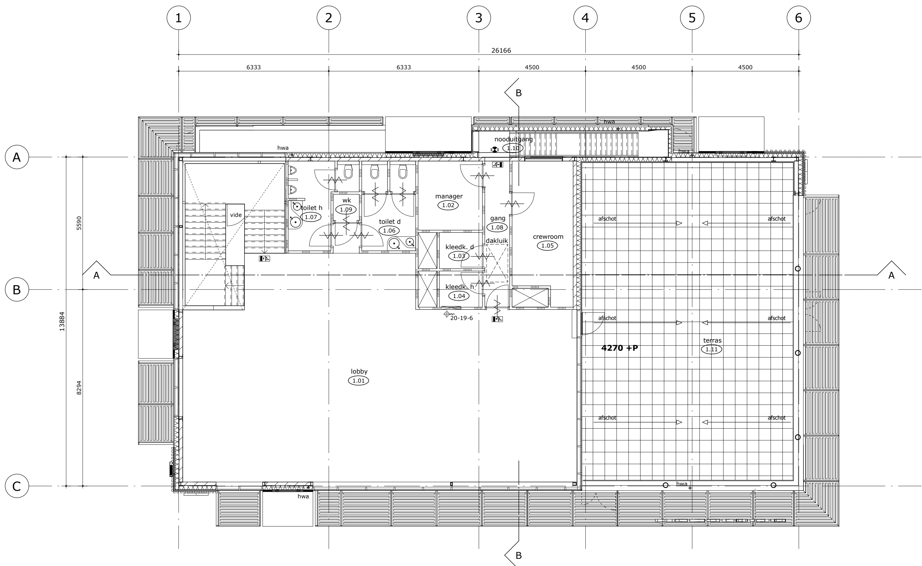
1e verdieping
