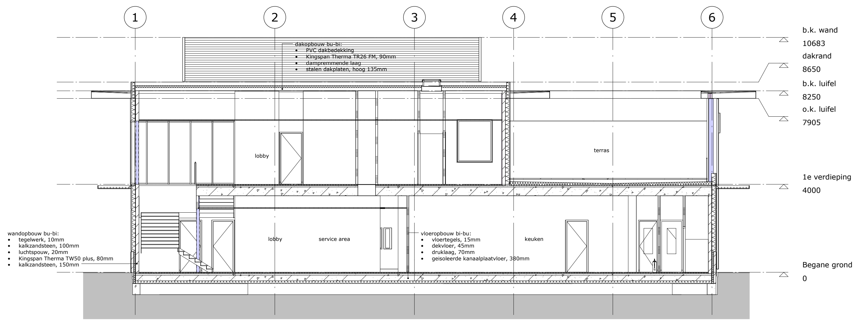
doorsnede A
