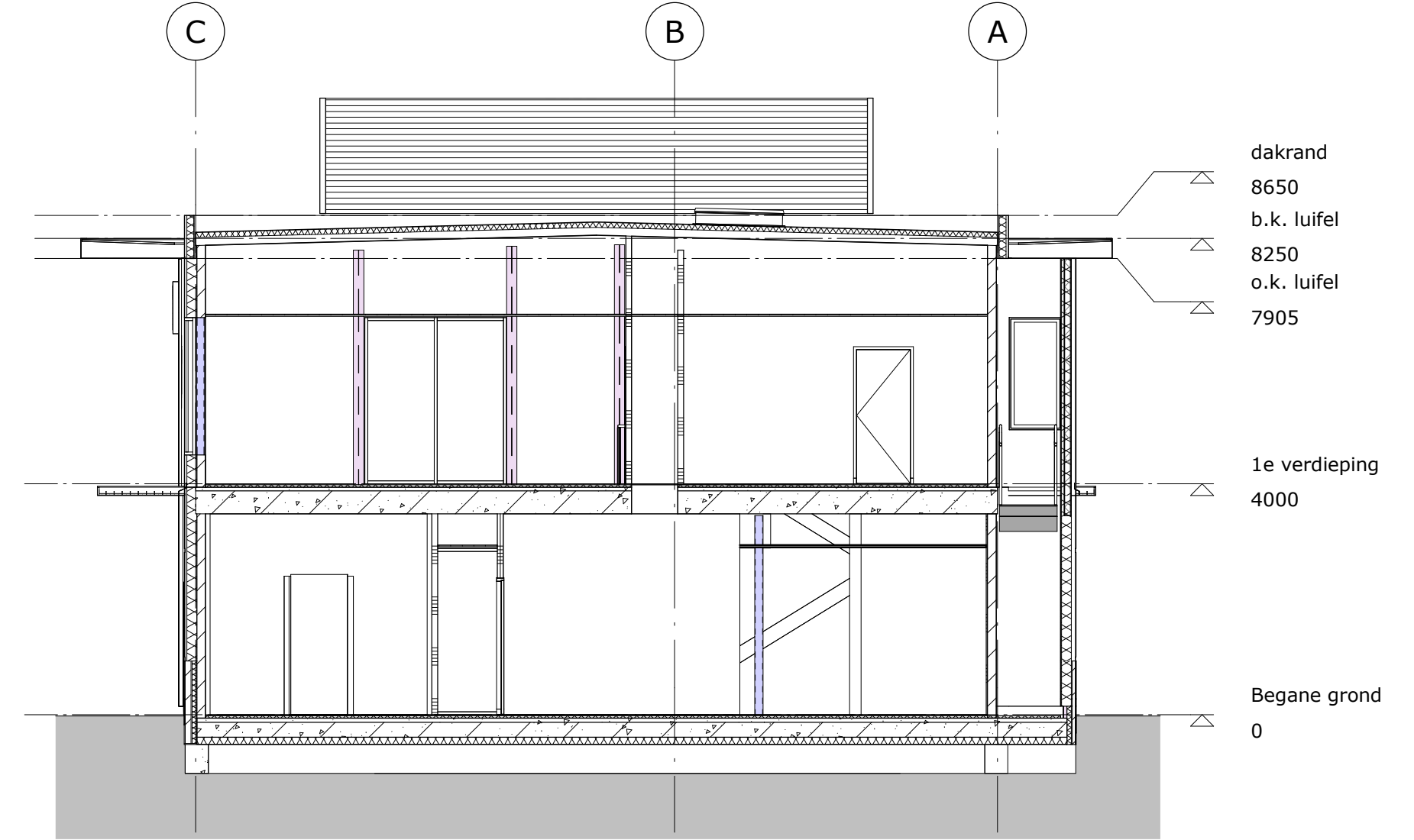
doorsnede B
