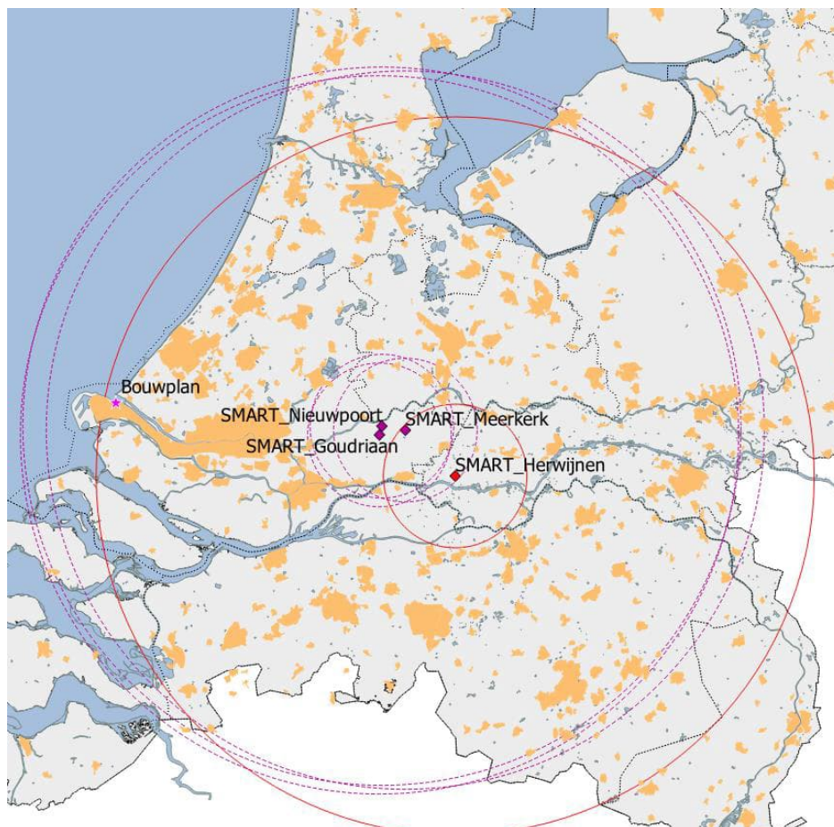
Figuur 5. Locaties van de drie alternatieve locaties Goudriaan, Meerkerk en Nieuwpoort (paarse ruit) voor de nieuwe SMART-L EWC GB gevechtsleidingsradar te Herwijnen (rode ruit). De oranje vlakken zijn de in de AHN-1 gedefinieerde stedelijke gebieden. De ligging van het te toetsen bouwplan is aangegeven met een roze ster.
