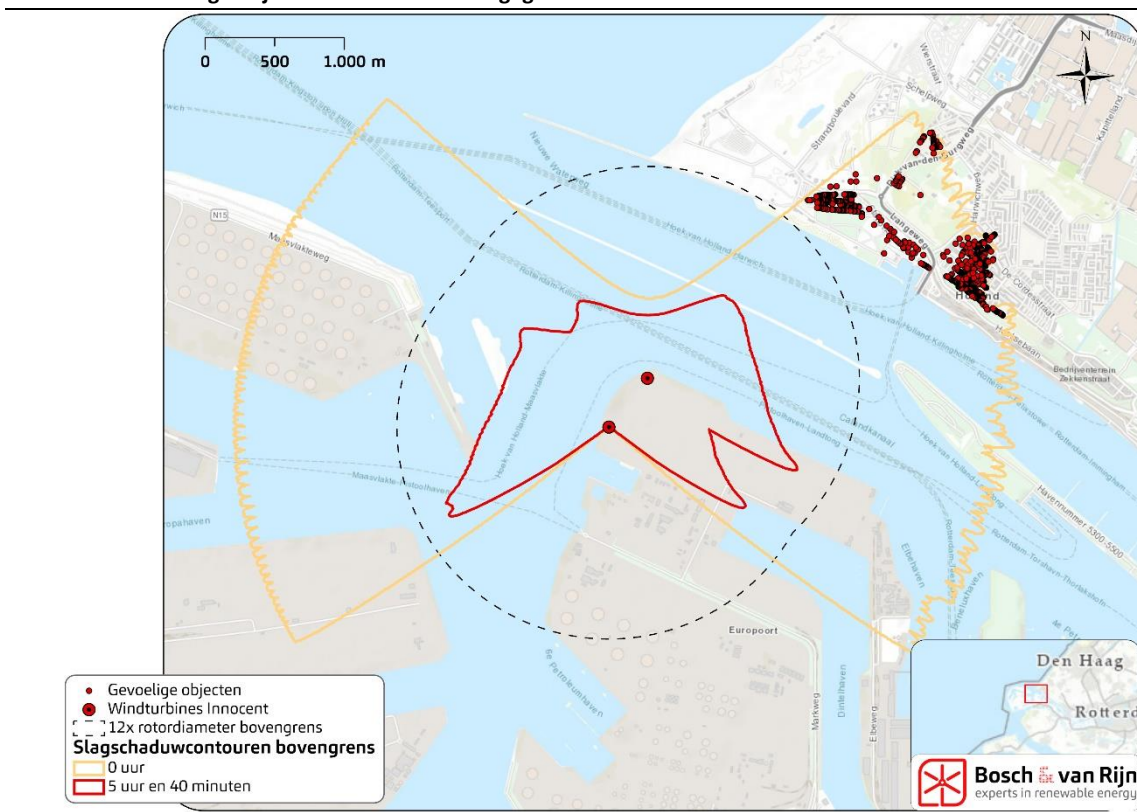
Figuur 5 De 5:40u en 0u slagschaduwcontouren van de bovengrens van de bandbreedte. Hierbij zijn ook gevoelige objecten van derden weergegeven.
