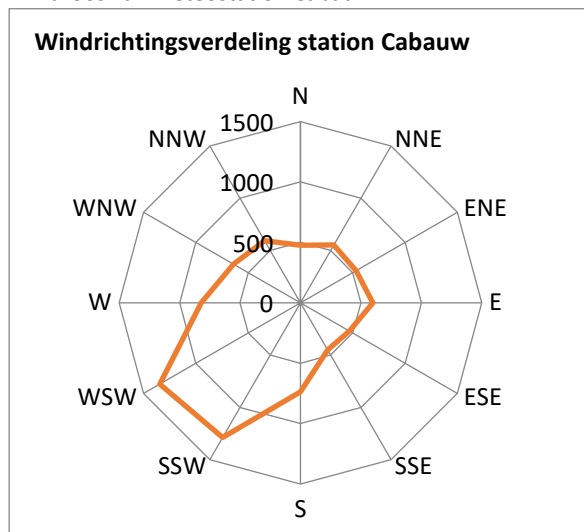
Figuur 3 Windroos van meteostation Cabauw.
