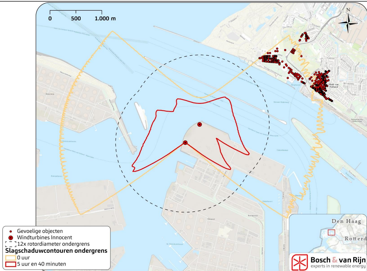
Figuur 8 De 5:40u en 0u slagschaduwcontouren van de ondergrens van de bandbreedte. Hierbij zijn ook gevoelige objecten van derden weergegeven.
