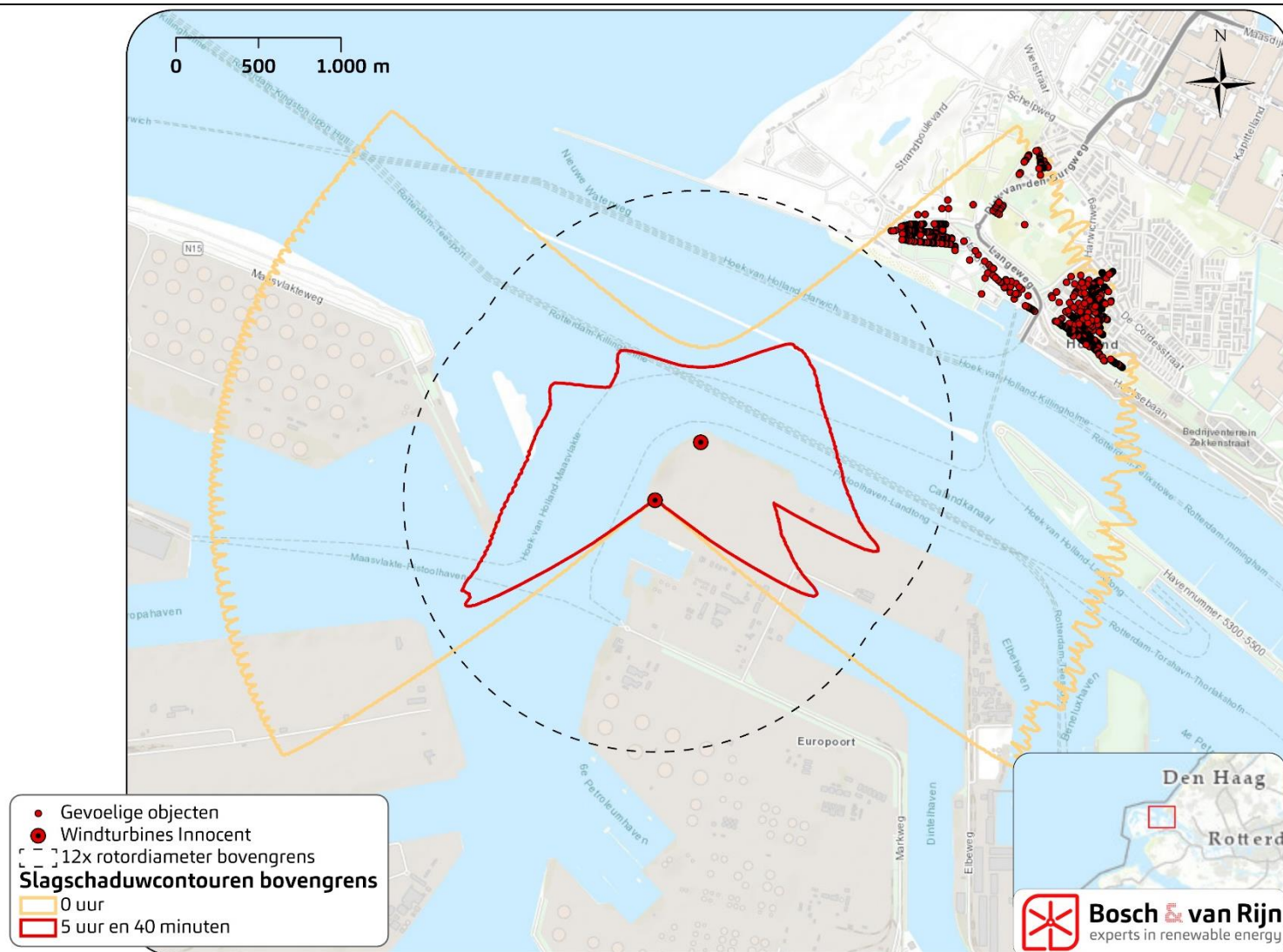
Figuur 9 De 5:40u en 0u slagschaduwcontouren van de bovengrens van de bandbreedte. Hierbij zijn ook gevoelige objecten van derden weergegeven.
