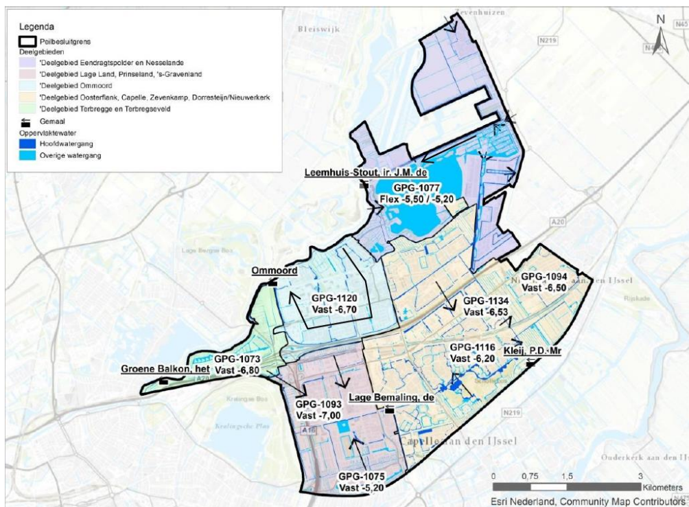
Figuur 7.3: Waterhuishouding in de Prins Alexanderpolder (bron: Peilbesluit Polder Prinseland en Eendragtpolder, HHSK, 2019)
