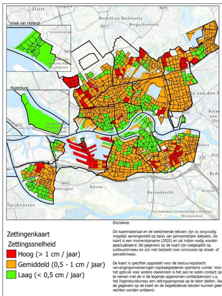
Figuur 5.3: Zettingenkaart
