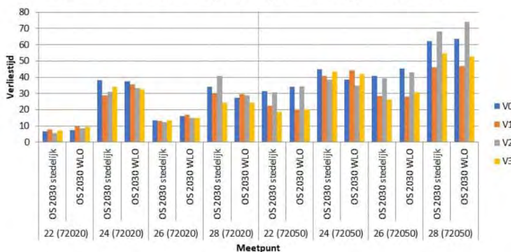
Figuur 10 Gemiddelde verliestijd fietsers ochtendspits
