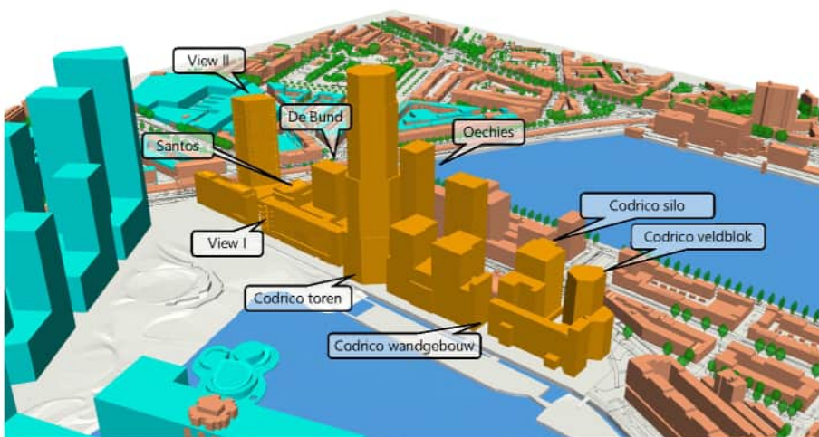
f 1.2 Het gehanteerde 3D-model van de plansituatie
