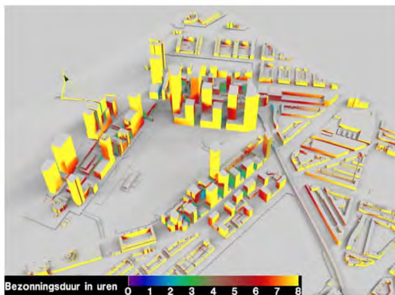
Bezonningsduur plansituatie 21 juni
