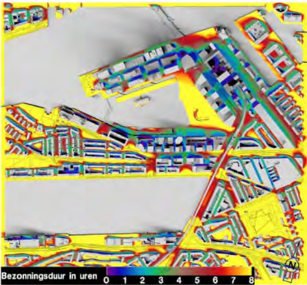
Bezonningsduur plansituatie 21 september
