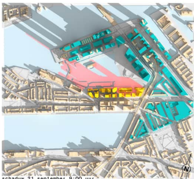
schaduw 21 september 9:00 uur
