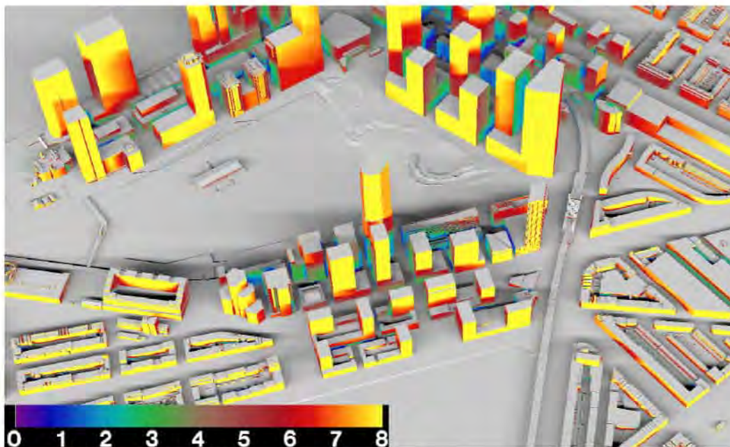
f 3.3 Bezonningsduur plansituatie op 21 september (zie ook bijlage 2)
