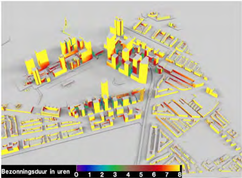
Bezonningsduur plansituatie 21 juni
