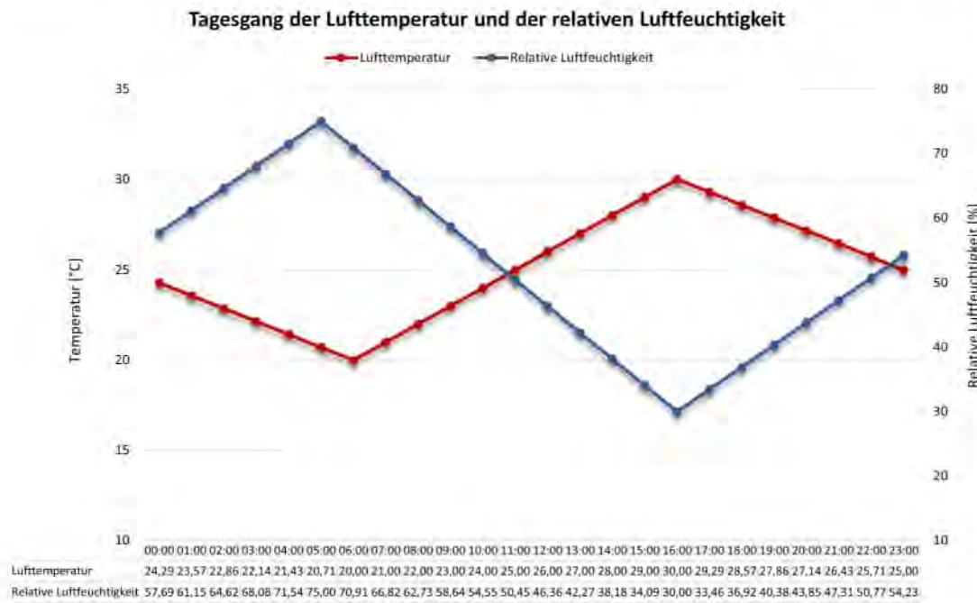
Abbildung 5.1: Tagesgang der Lufttemperatur und der relativen Luftfeuchtigkeit beim Simple-Forcing
