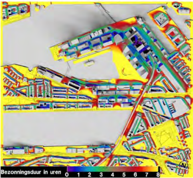
Bezonningsduur referentiesituatie 21 september
