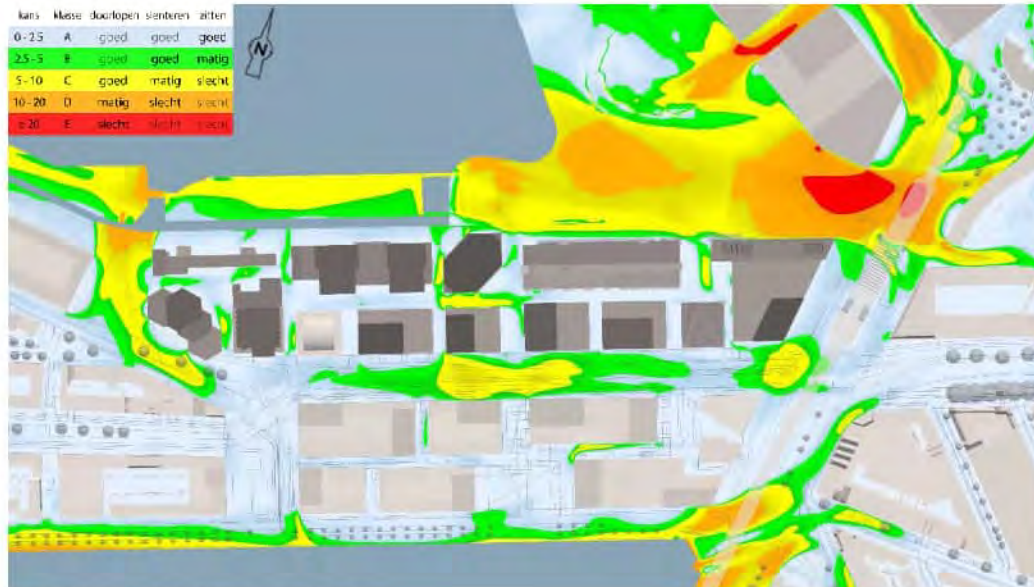
f 5.2 Windhinder in de toekomstige situatie
