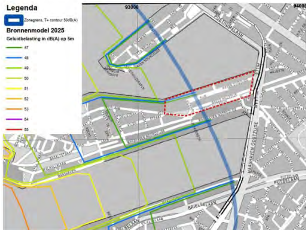
F 14 Geluidcontouren Bronnenmodel 2025
