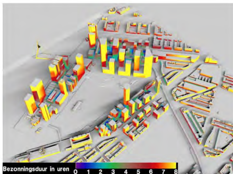
Bezonningsduur plansituatie 21 september
