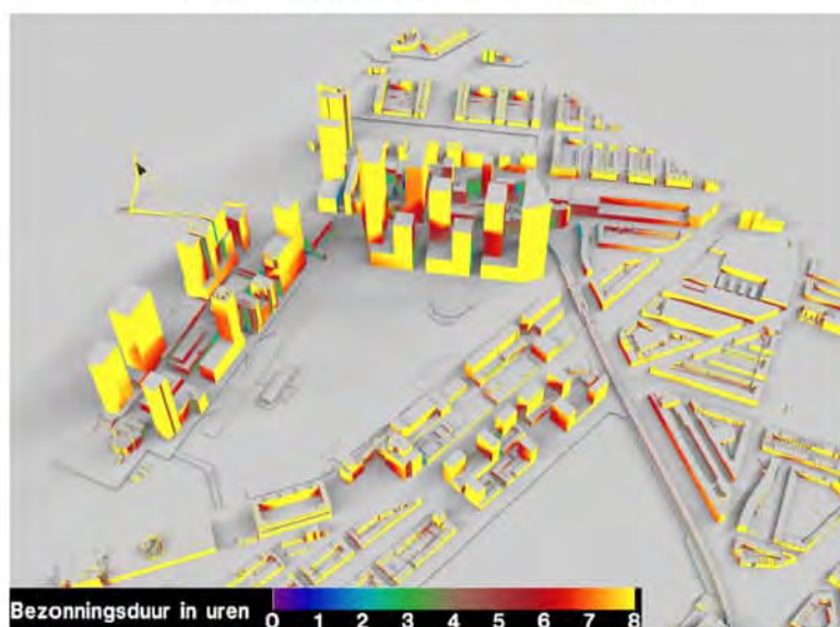
Bezonningsduur referentiesituatie 21 juni
