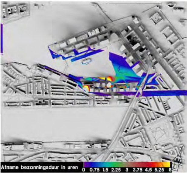
Afname bezonningsduur 21 september
