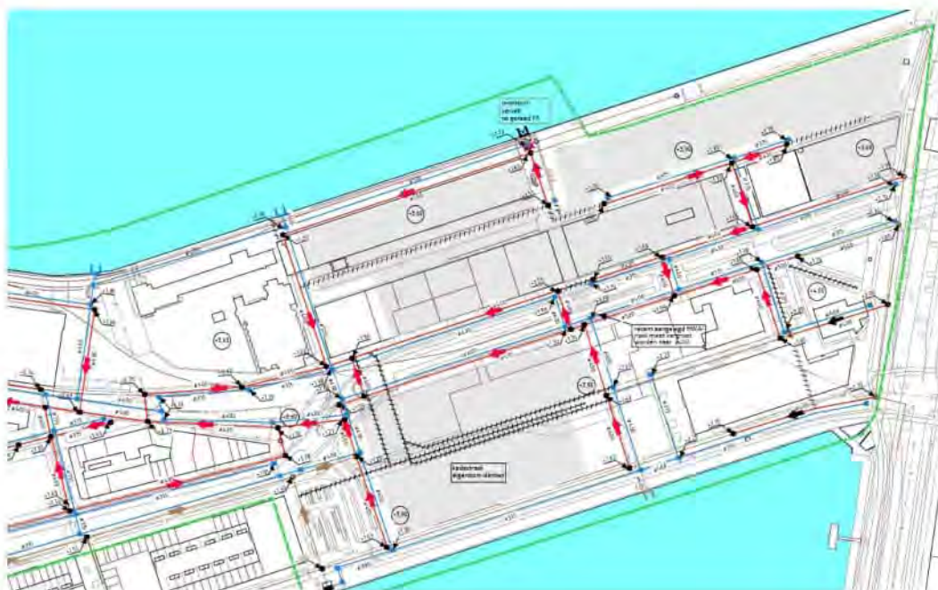
F 35 Basisontwerp riolering Katendrecht
