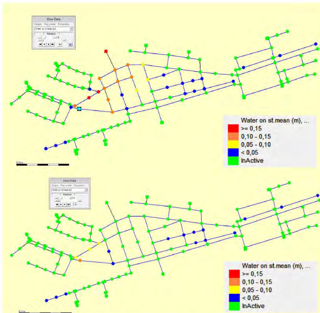
Figuur 9 Water-op straat bui 09: boven zonder uitlaat Linker Veerdam, onder met uitlaat Linker Veerdam
