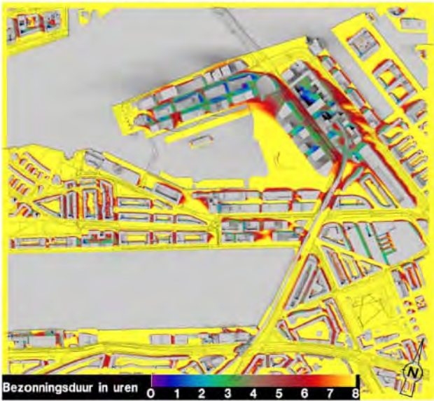
Bezonningsduur referentiesituatie 21 juni
