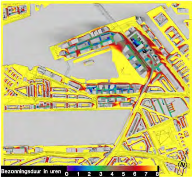
Bezonningsduur plansituatie 21 juni
