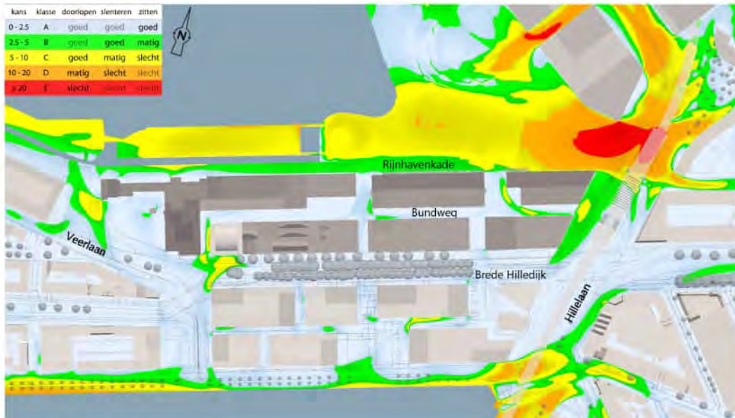
f 3.2 Windhinder in de referentiesituatie
