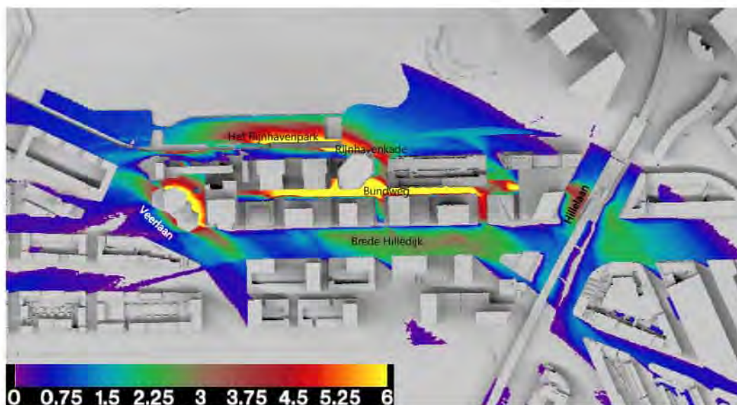
f 3.5 Afname bezonning op 21 juni (zie ook bijlage 3)
