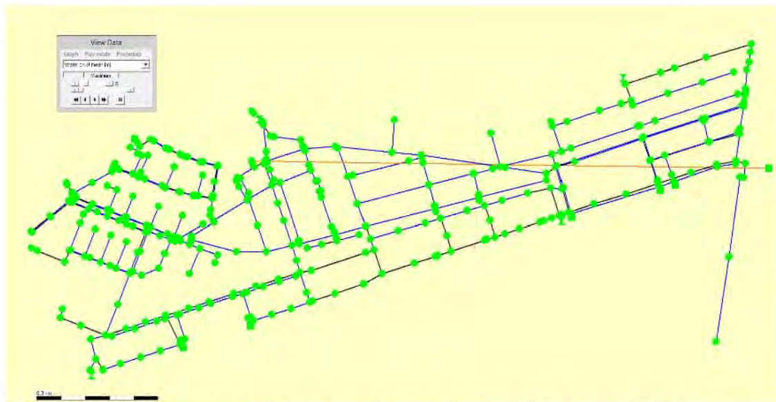
Figuur 14 Bui 08 DWA/gemengd stelsel na uitvoering Veerlaan, Siloplein en De Pols
