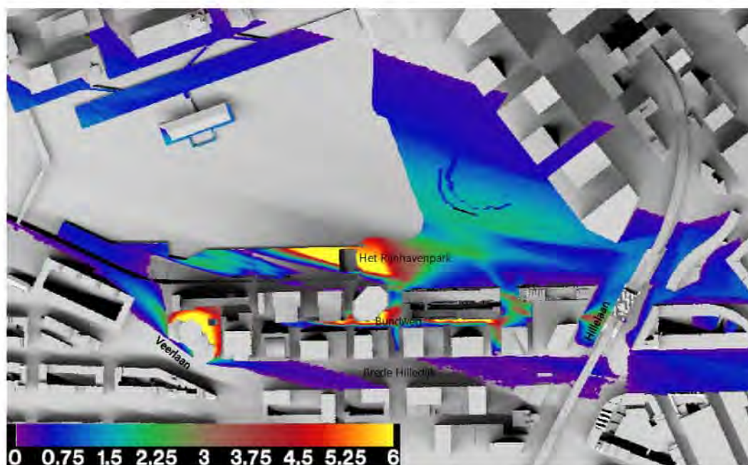
f 3.6 Afname bezonning op 21 september
