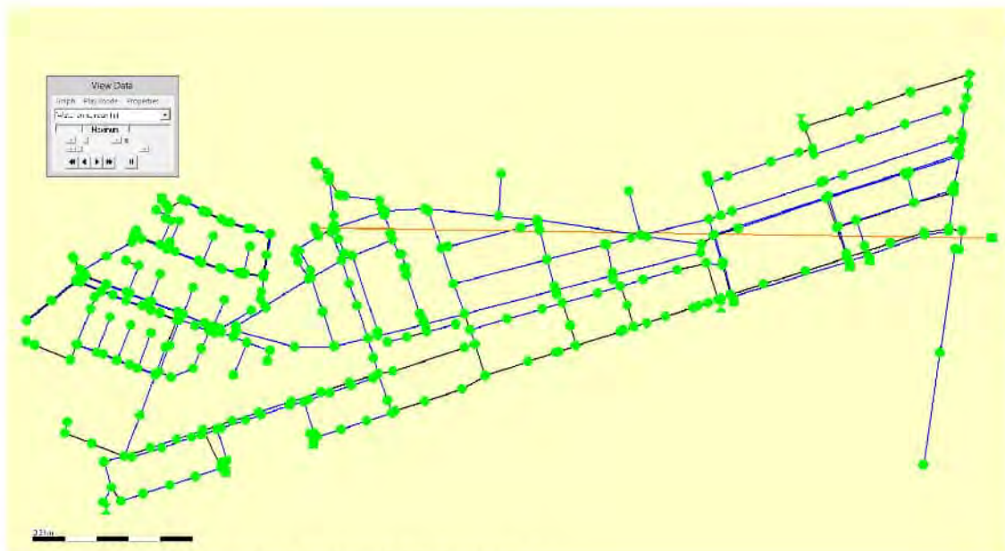
Figuur 7 DWA/gemengd stelsel eindsituatie bui 08
