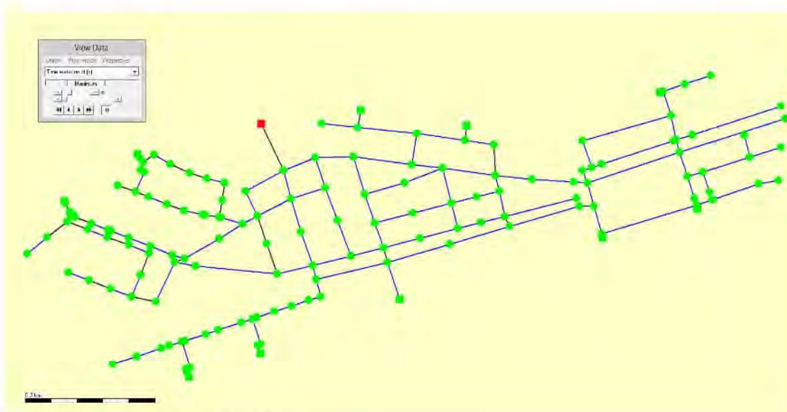
Figuur 6 HWA eindsituatie bui 08
