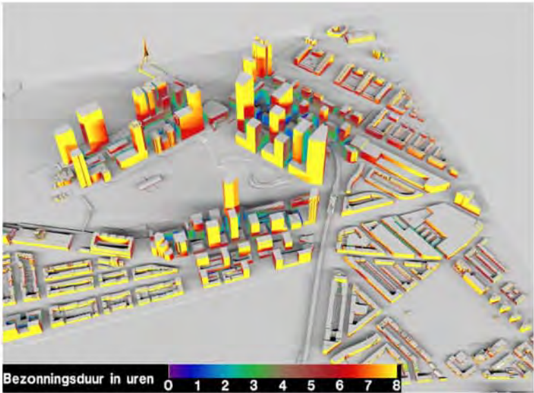
Bezonningsduur plansituatie 21 september
