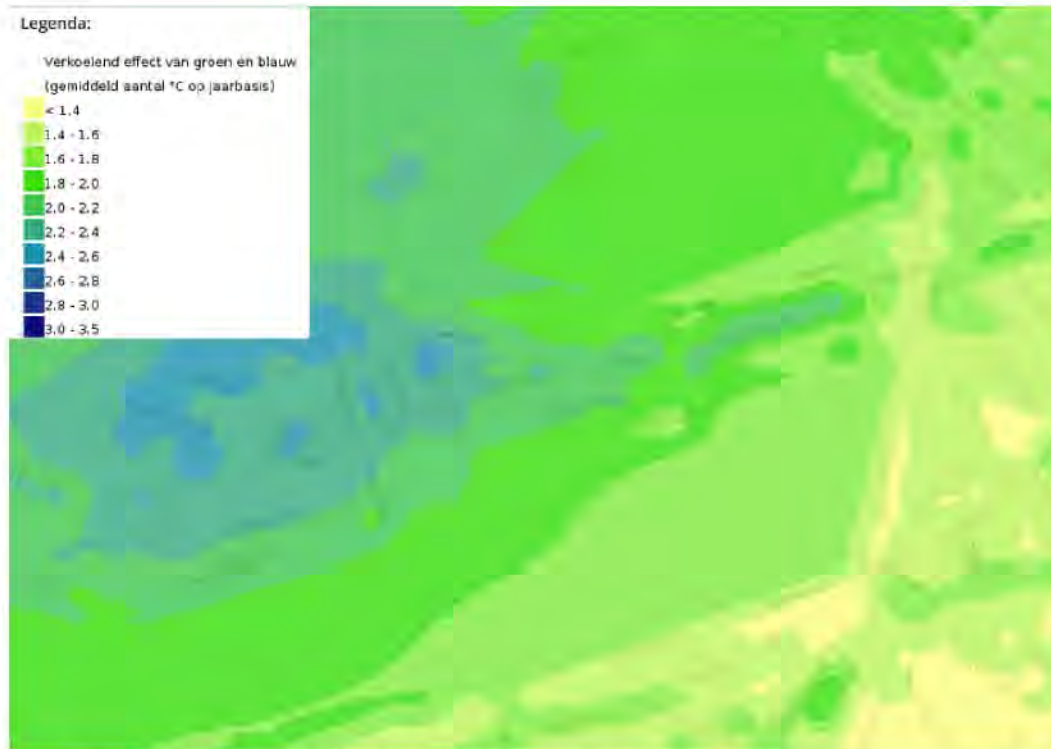
F 26 Kaart verkoelend effect groen en water (bron: Atlas Leefomgeving)
