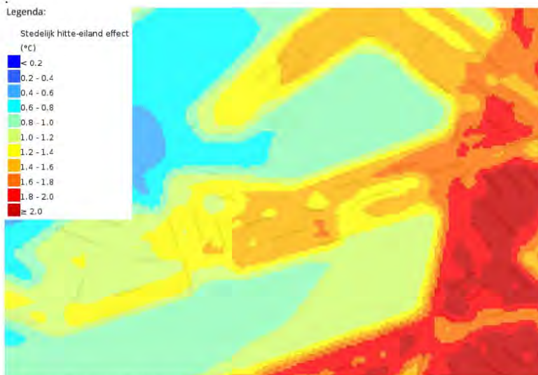
F 25 Hittestress kaart (bron: Atlas Leefomgeving)
