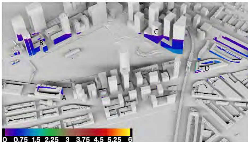
f 3.4 Afname bezonning op 21 september (zie ook bijlage 2)
