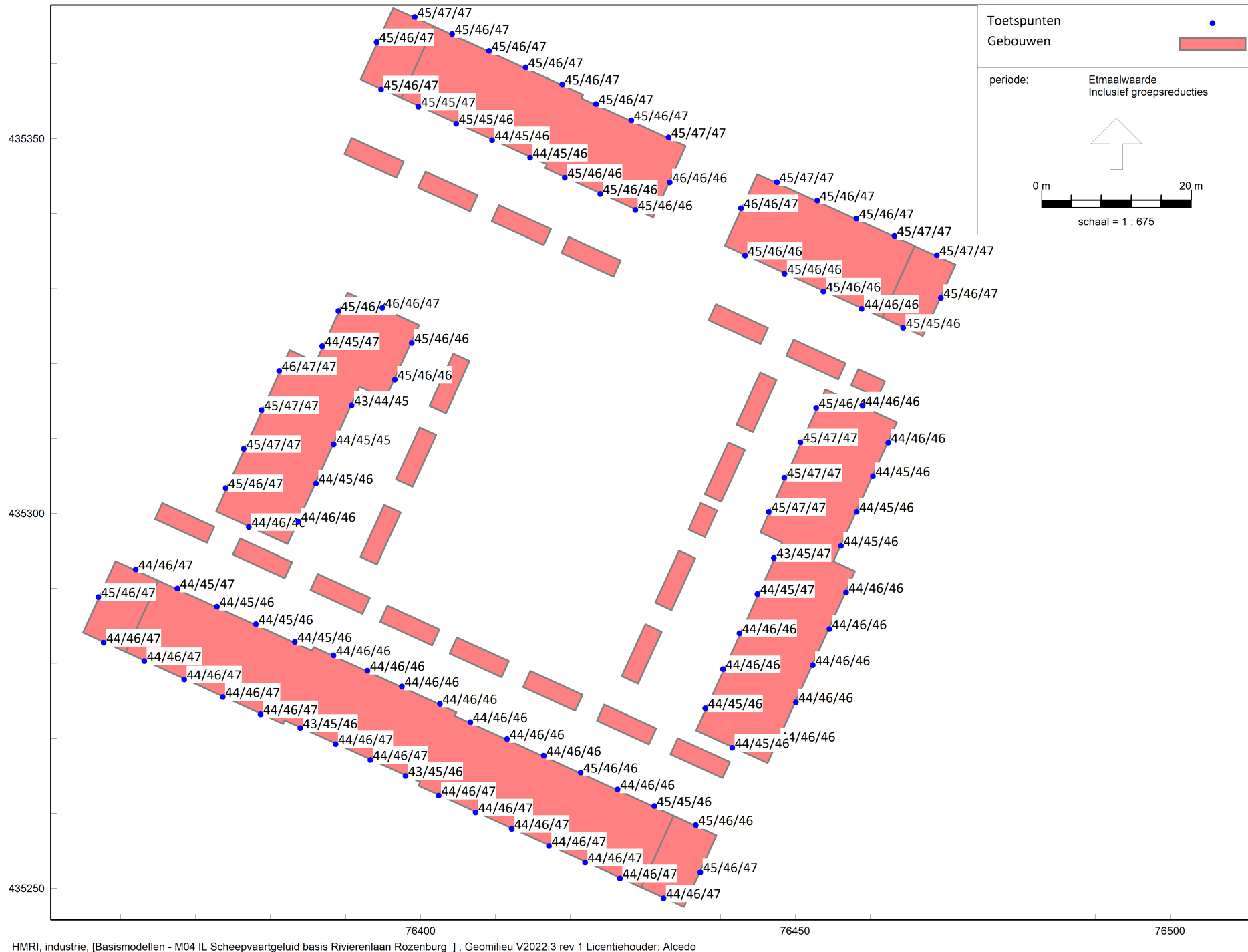
Figuur 13 Rekenresultaten Scheepvaartgeluid
