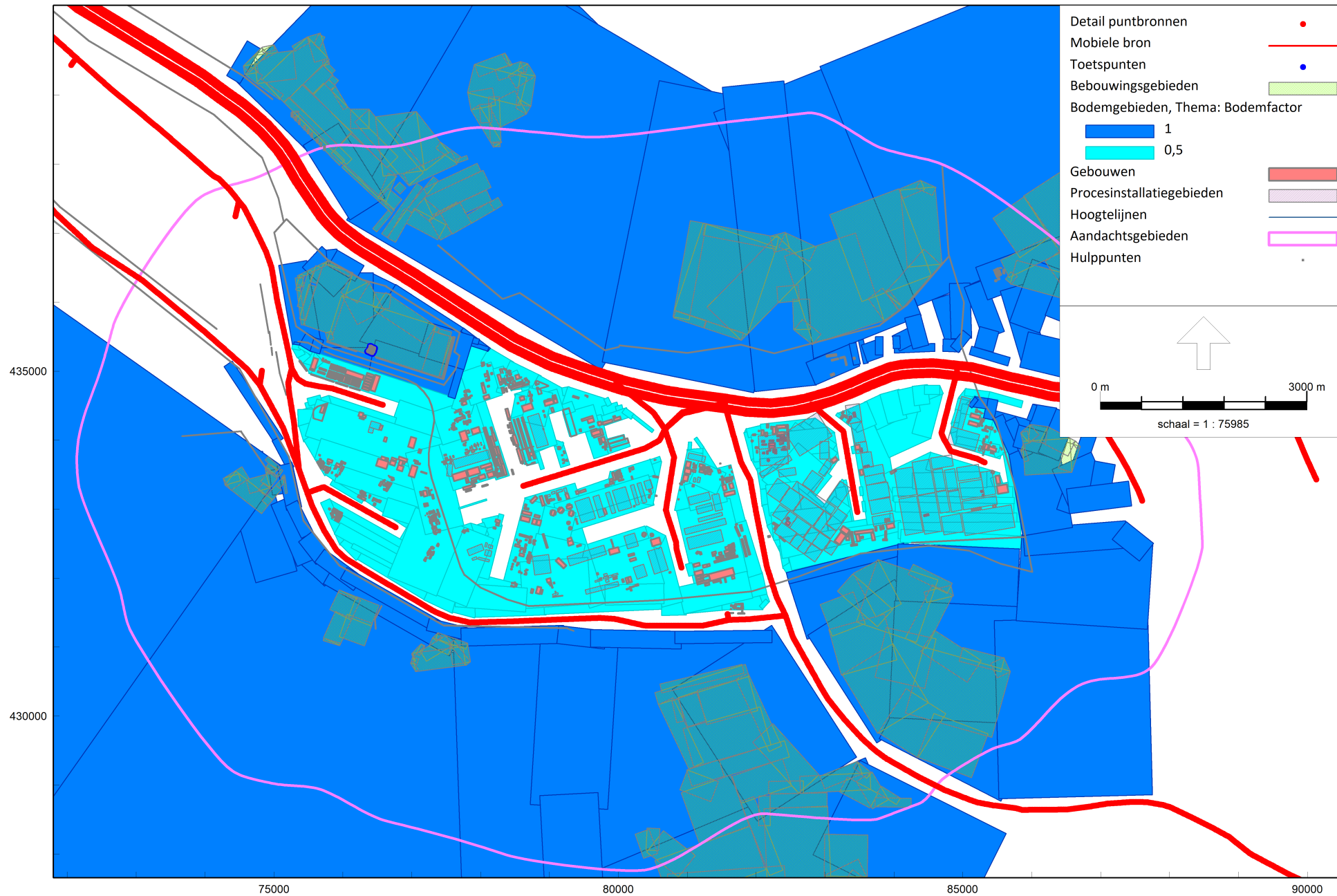
Figuur 7 Overzicht rekenmodel scheepvaartgeluid
