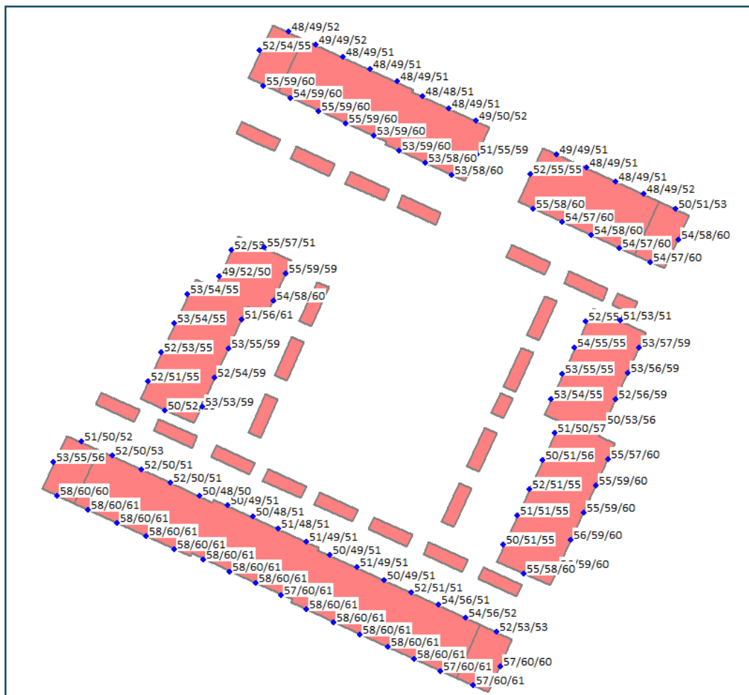
Figuur 12 Berekende geluidbelasting ter plaatse van de planlocatie vanwege Botlek-Pernis
