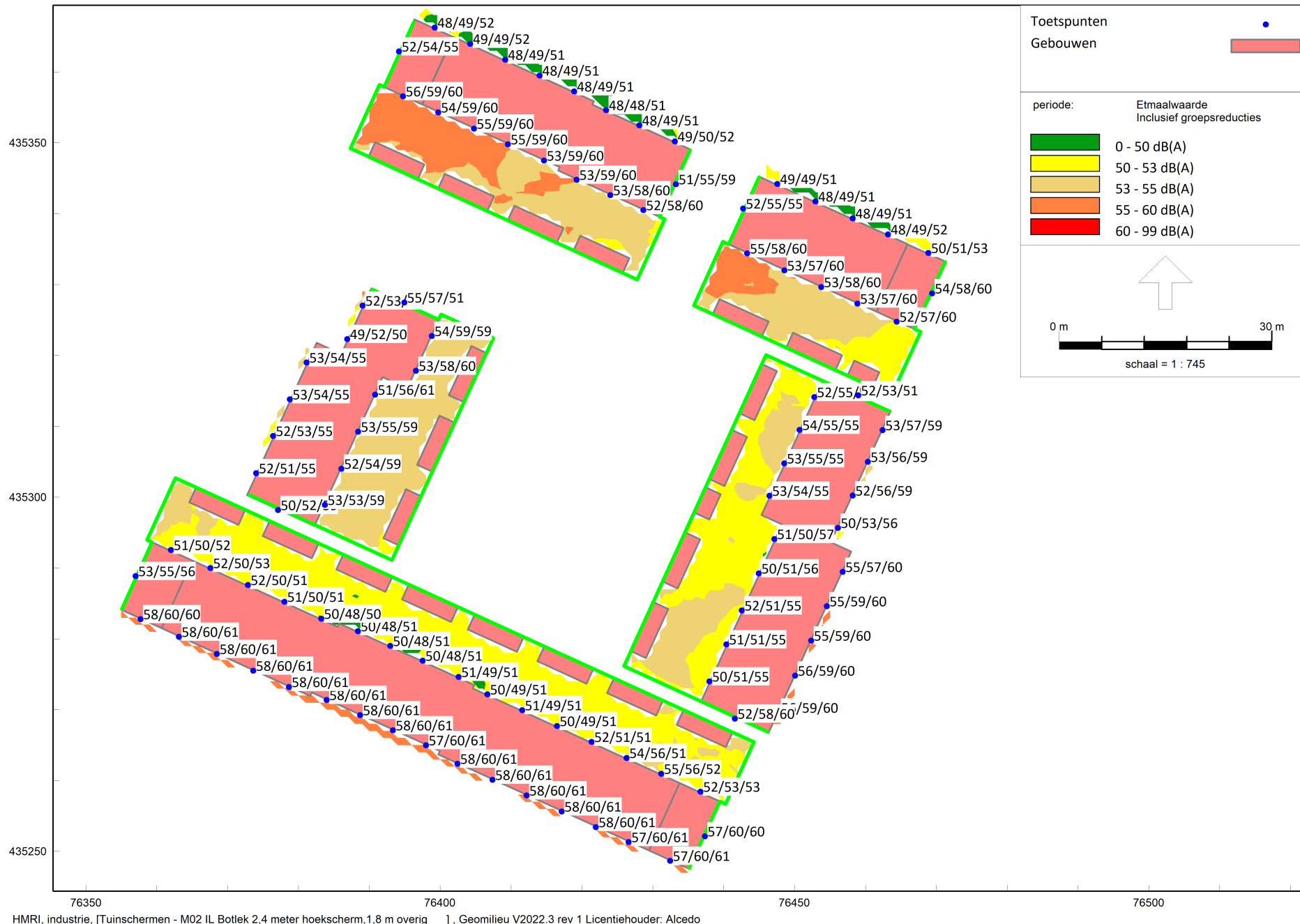
Figuur 14 Rekenresultaten voor Botlek-Pernis, met 2,4 meter hoekscherf en 1,8 meter overig inclusief contouren tuinen op 1,2 meter
