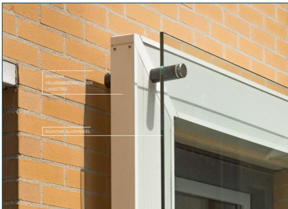
Figuur 19 Plaat glas aan de buitenzijde voor een draaiend deel met absorberende cassettes langs de randen
