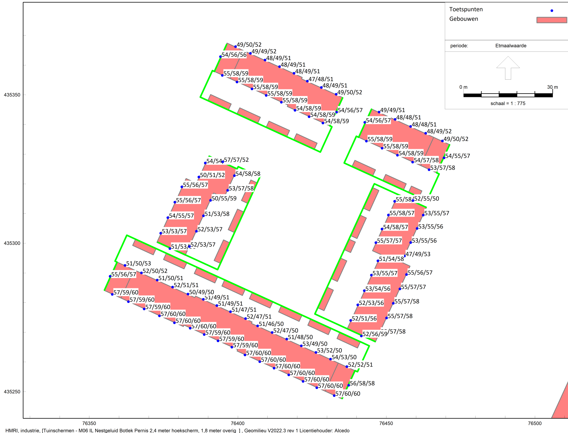
Figuur 15 Rekenresultaten nestgeluid Botlek-Pernis met schermen
