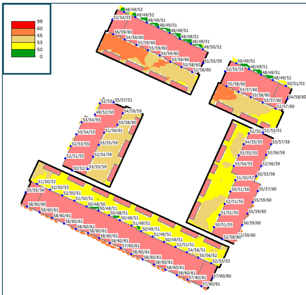
Figuur 18 Resultaten na het toepassen van tuinafsluiting (contouren op een hoogte van 1,2 meter en puntresultaten op een hoogte van 1,5/4,5 en 7,5 meter hoogte)
