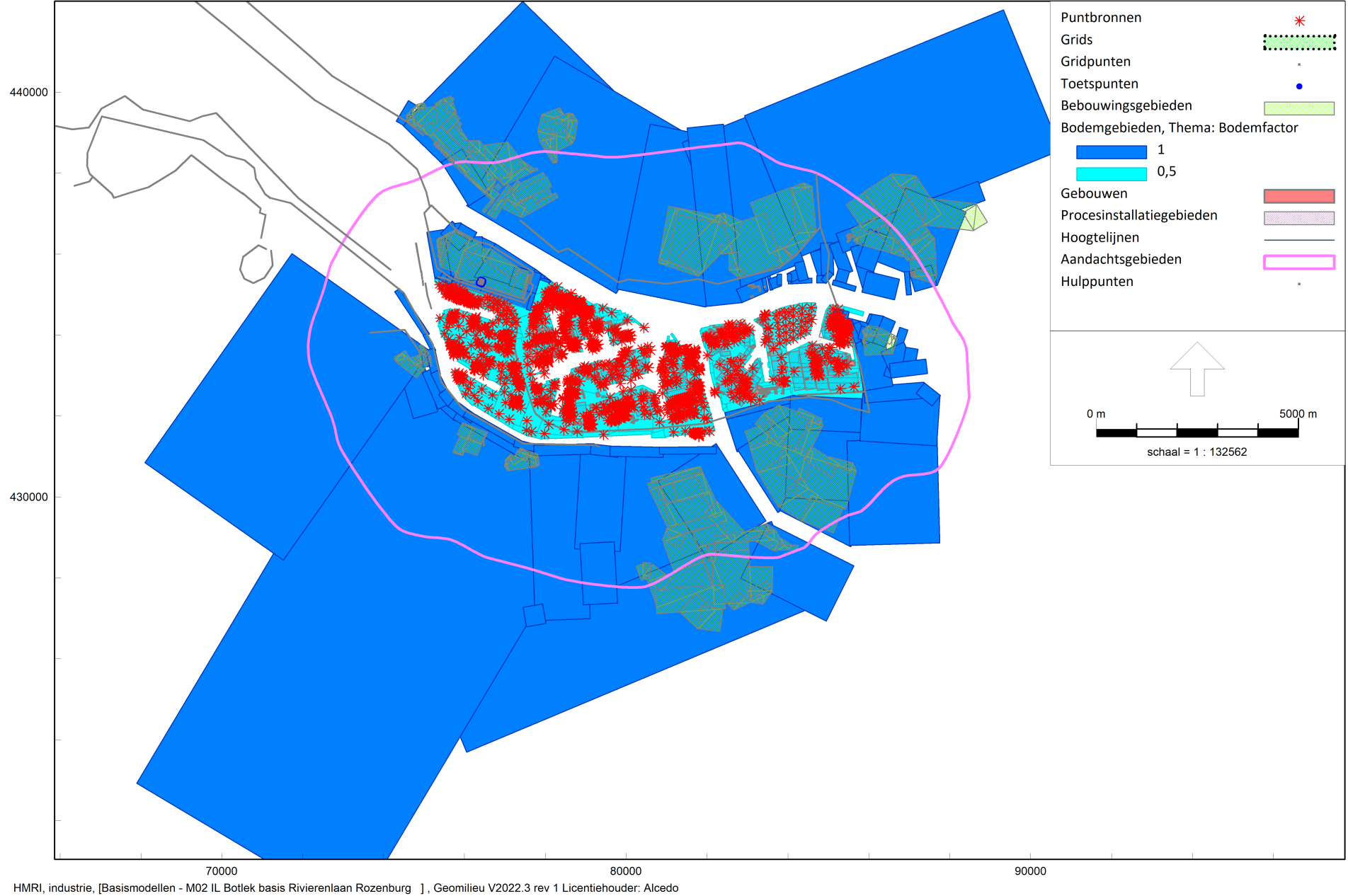
Figuur 4 Overzicht rekenmodel Botlek
