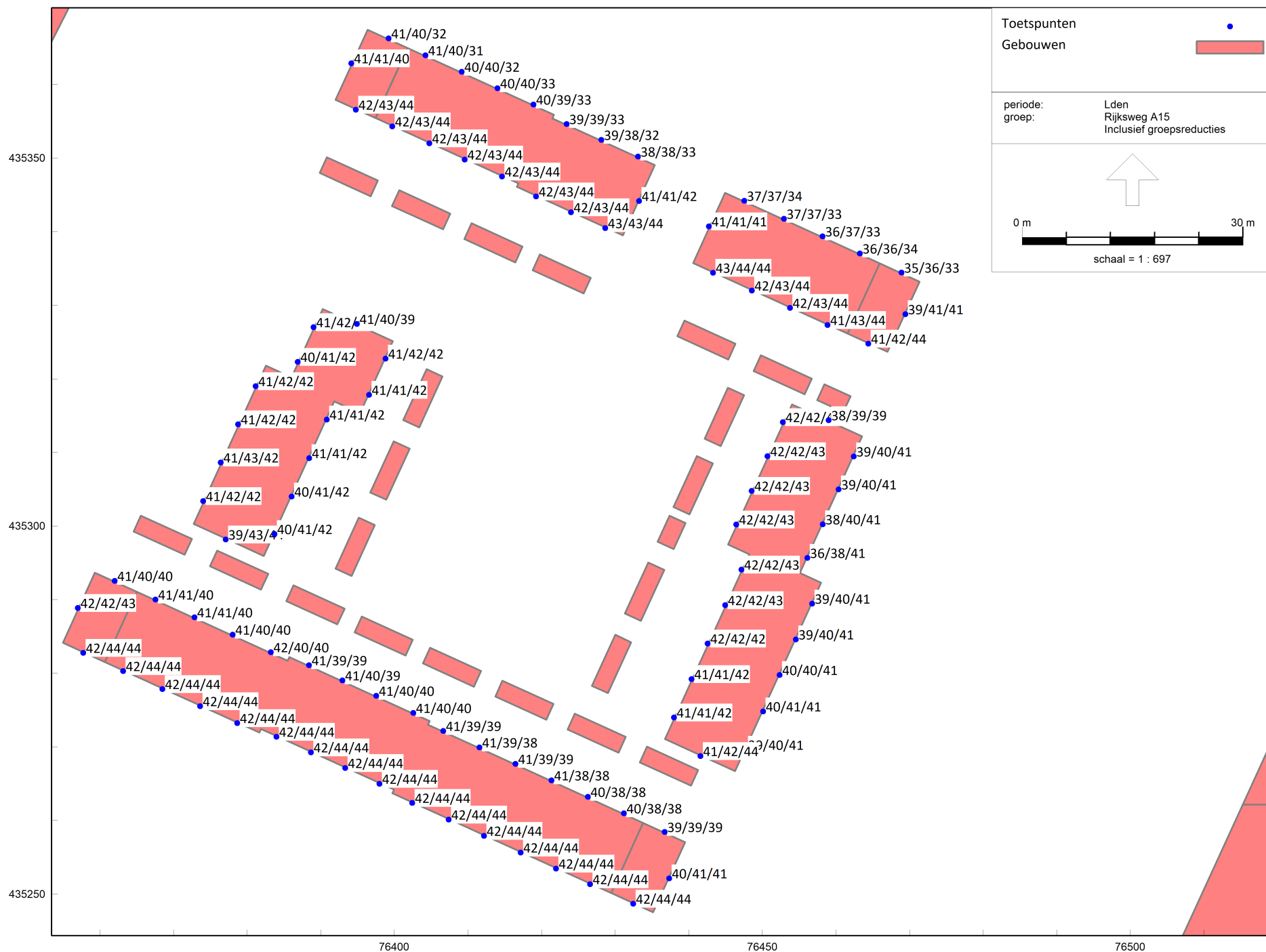
Figuur8 Rekenresultaten Rijksweg A15 inclusief 2 dB correctie
