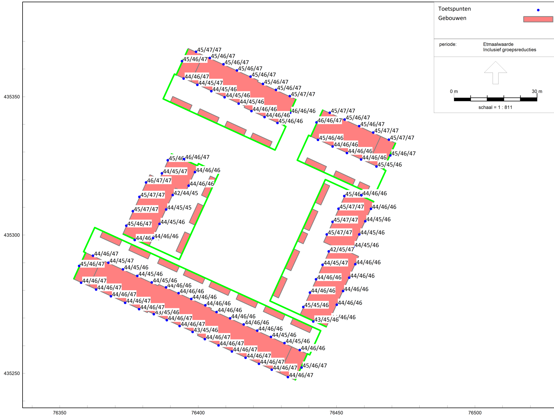
Figuur 17 Scheepvaartgeluid met schermen
