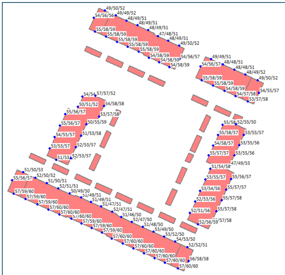
Figuur 14 Berekende geluidbelasting ter plaatse van de planlocatie vanwege nestgeluid van Botlek-Pernis
