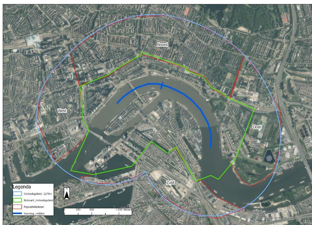
figuur B1.1: ligging vaarweg, invloedsgebied, en blokken. Het streepje door de vaarweg is de scheiding tussen het brede en smalle deel van de vaarweg.
