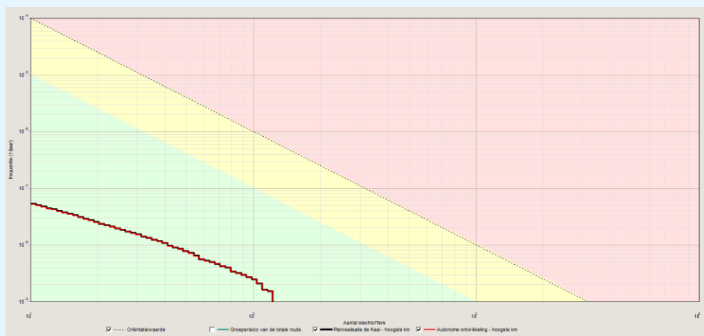
figuur 4: fN-curve autonoom (rood) en planrealisatie (zwart). De curves liggen vrijwel over elkaar.
