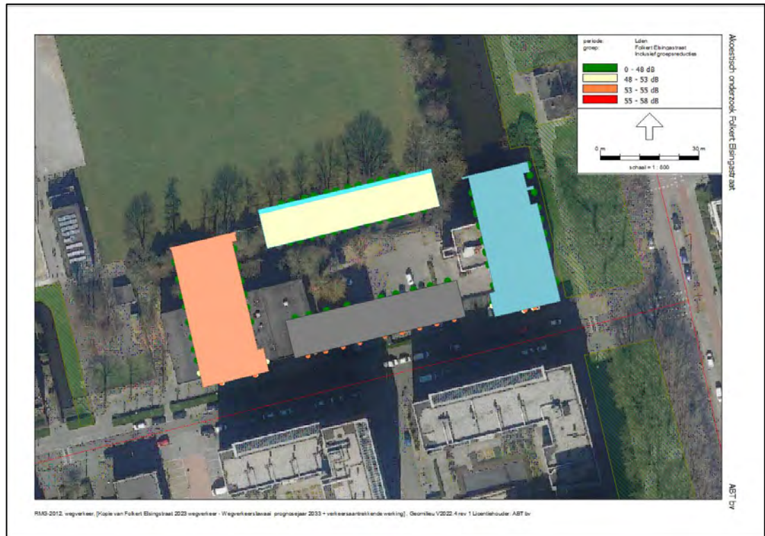
Afbeelding 3 L_{den} dB Folkert Elsingastraat
