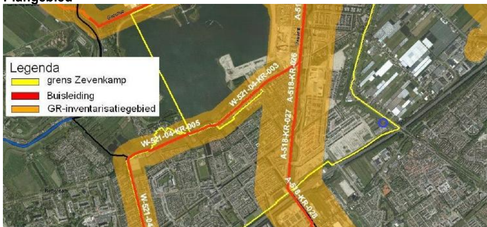
Figuur 13 - Ligging gasleidingen met planlocatie (blauw omcirkeld). Bron: DCMR
