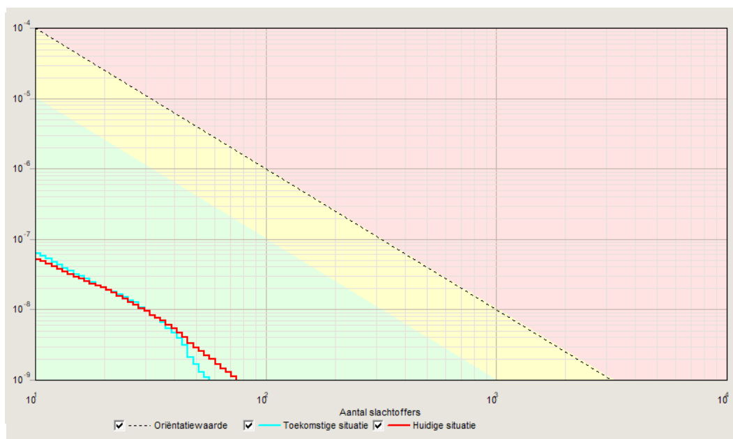
f5.2 Berekende fN-curves voor de huidige situatie (rood) en toekomstige situatie (blauw)
