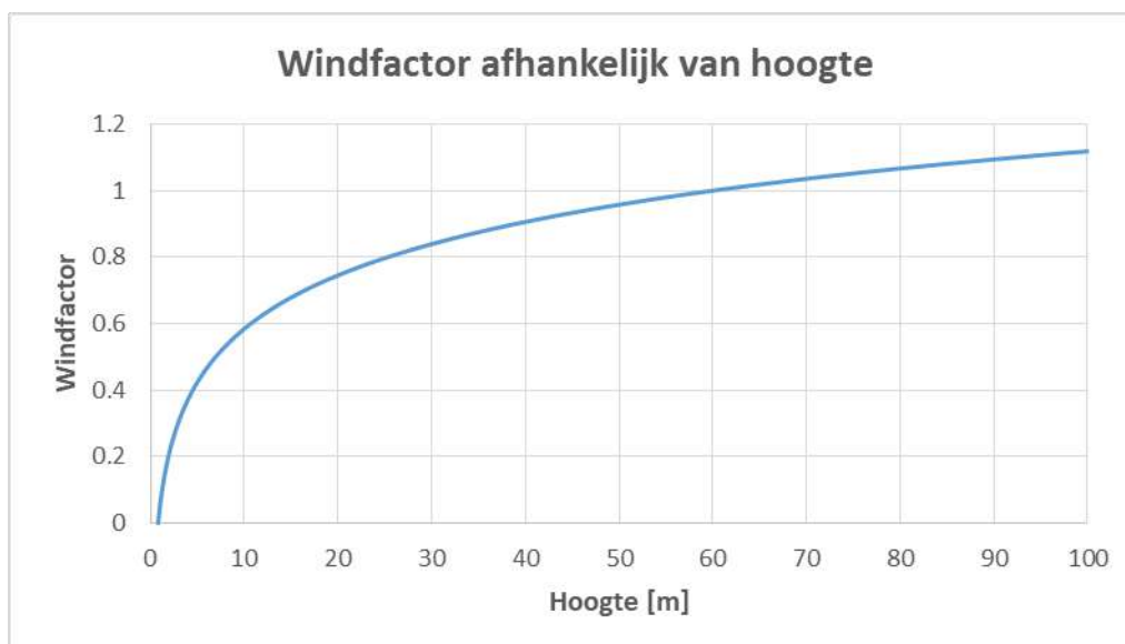
Figuur 5: Toegepast windprofiel met referentiehoogte op 60 meter.
