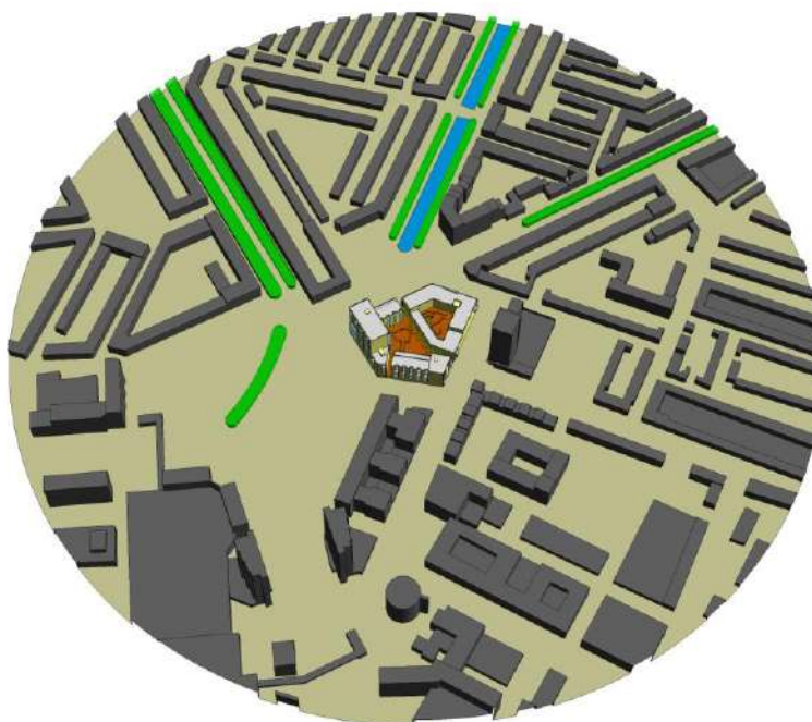
Figuur 1: Overzicht van het 3D CFD model met omliggende bebouwing.
