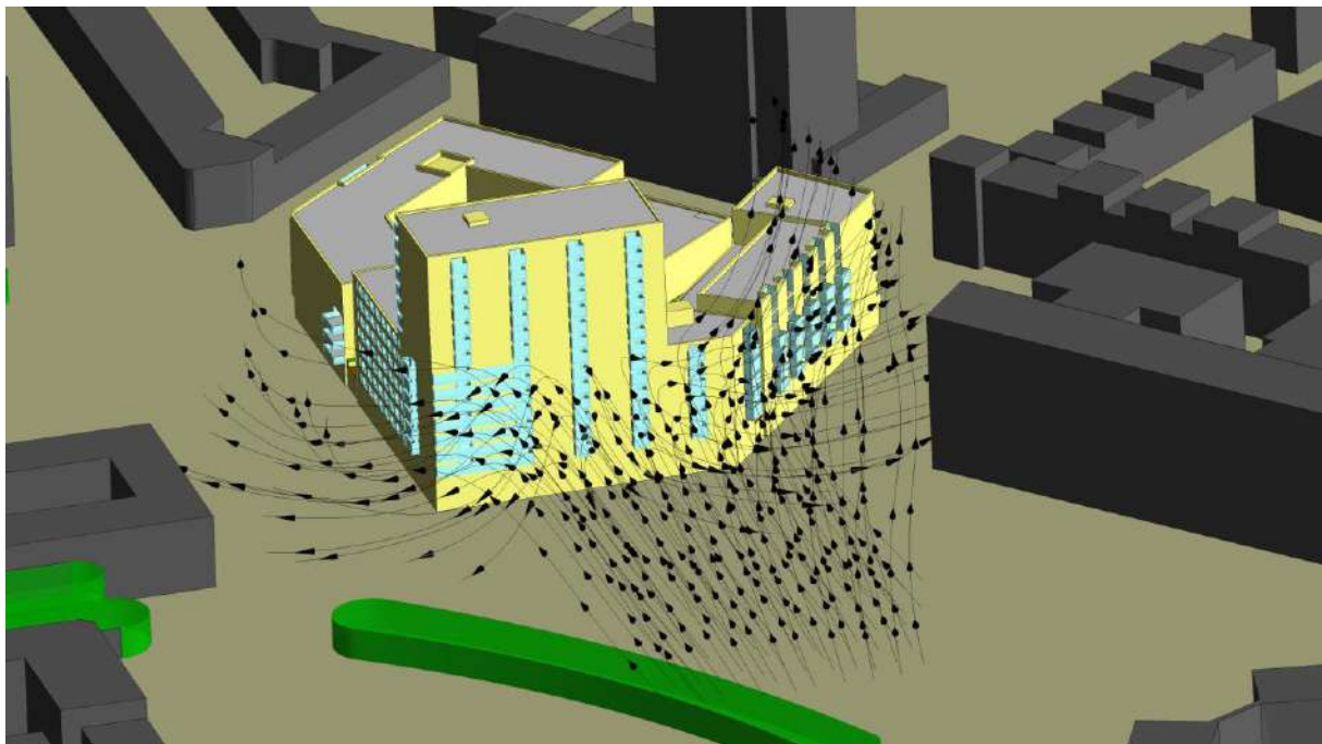
Figuur 10: 3D weergaven van de luchtstroom om de nieuwbouwontwikkeling bij windrichting west (270 graden).
