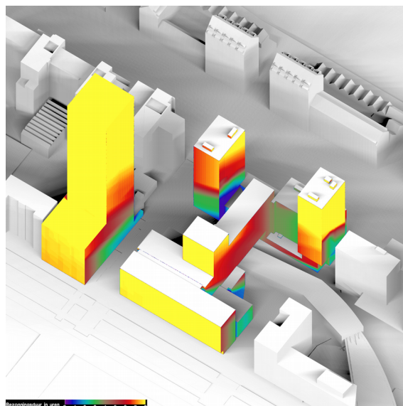
Bezonningsduur bestaande situatie 21 september
