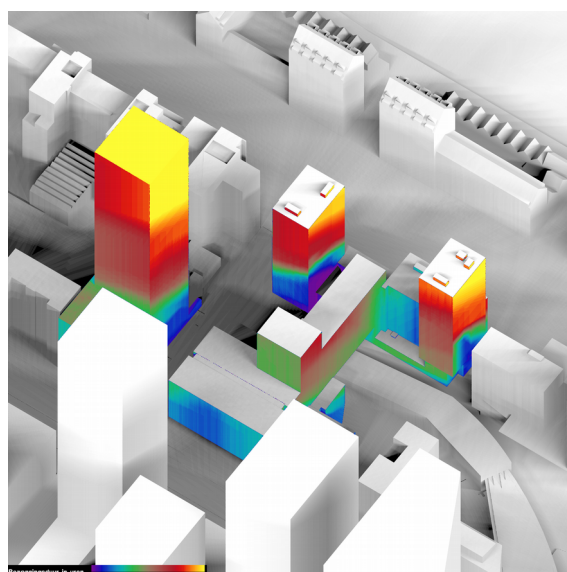
Bezonningsduur geplande situatie 21 september
