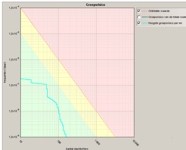
Figuur 2.1 groepsrisicocurve
