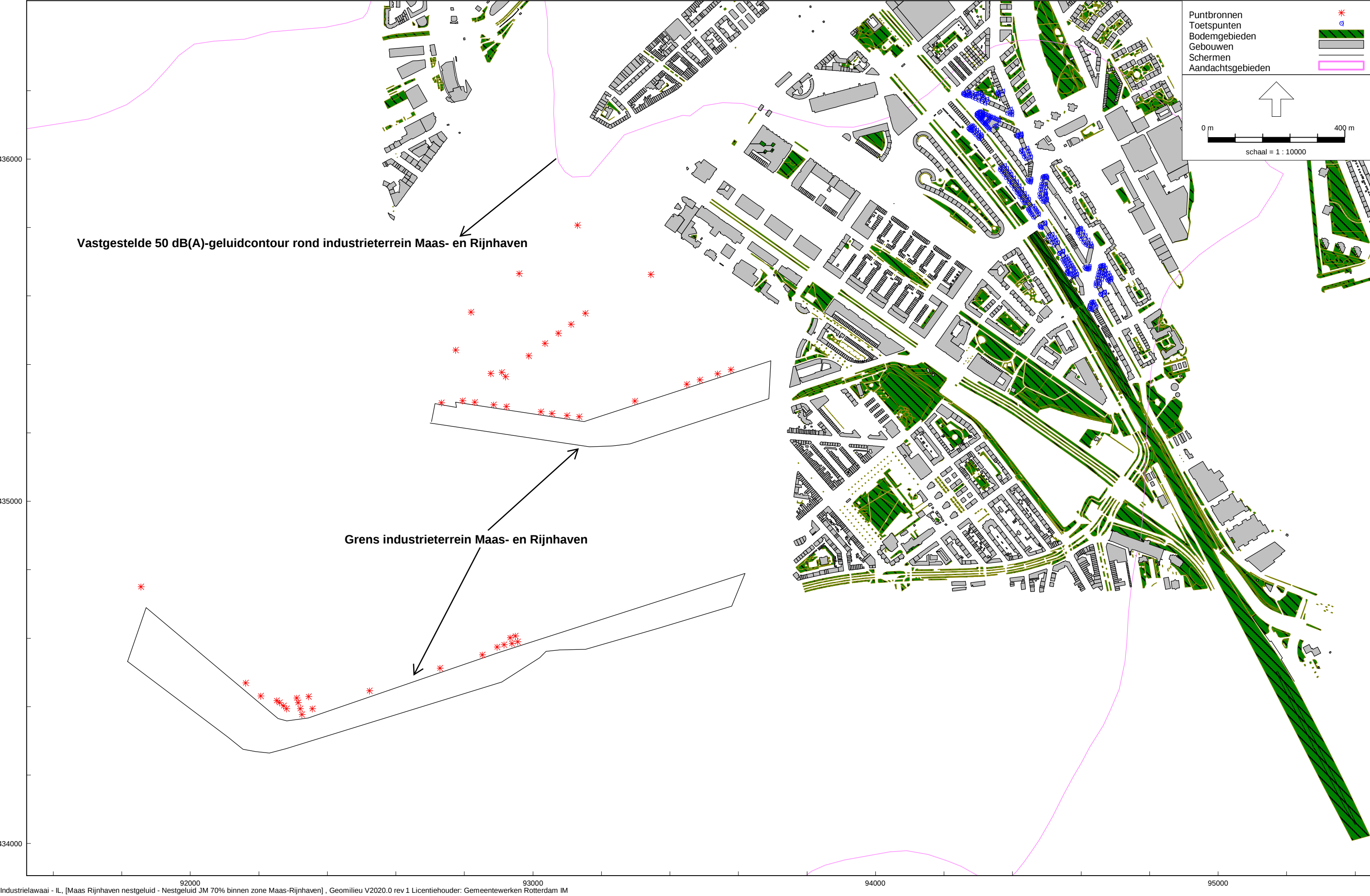
Bijlage 2a: Overzicht rekenmodel Nestgeluid (obv 70% jaargemiddelde ligplaatsbezetting) afkomstig van afgemeerde schepen in Maas- en Rijnhaven tbv bestemmingsplan Feijenoord
