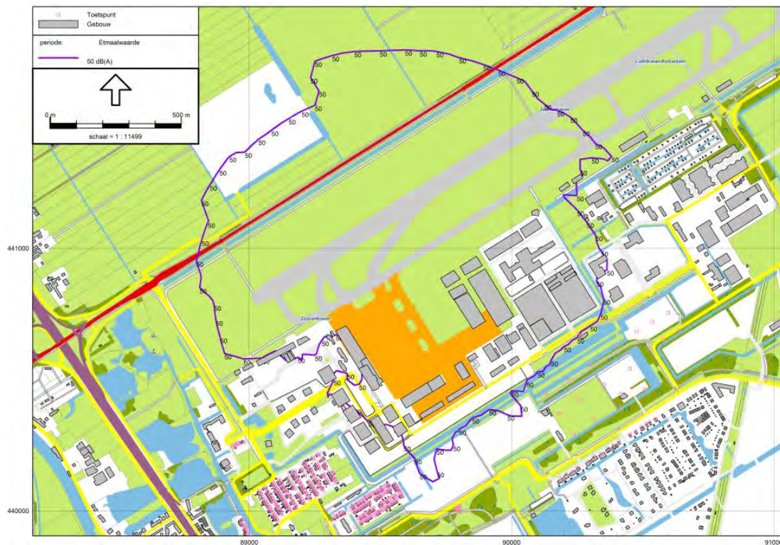
Figuur 16 Berekende 50 dB(A) L_{etmaal} -contour (paars) ten gevolge van de industrie (alleen het gezoneerde industrieterrein) in de plansituatie op basis van milieuzonering uit het bestemmingsplan.
