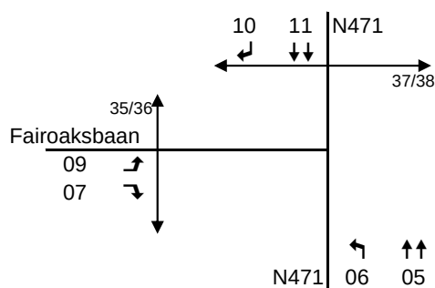
Figuur B3.4: Huidige vormgeving kruispunt 3
