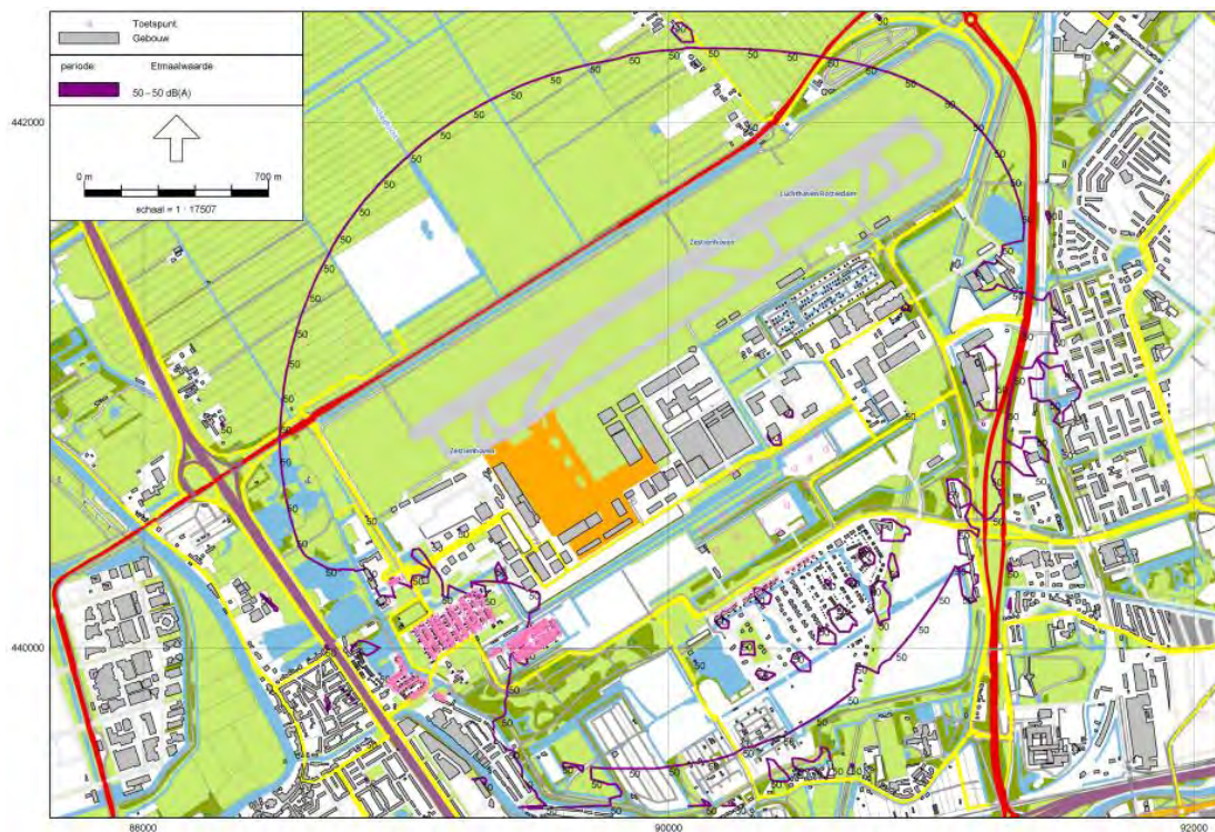
Figuur 21 50 dB(A) Letmaal-contour op basis van industrielawaai ten gevolge van proefdraaien, huidige vergunningen en maximale milieucategorieën uit het Masterplan.
