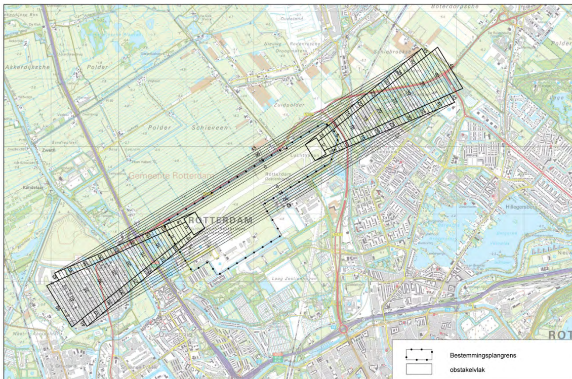
Figuur 9.1 Obstakelvrije vlakken (ten opzichte van NAP-4,4 m)
