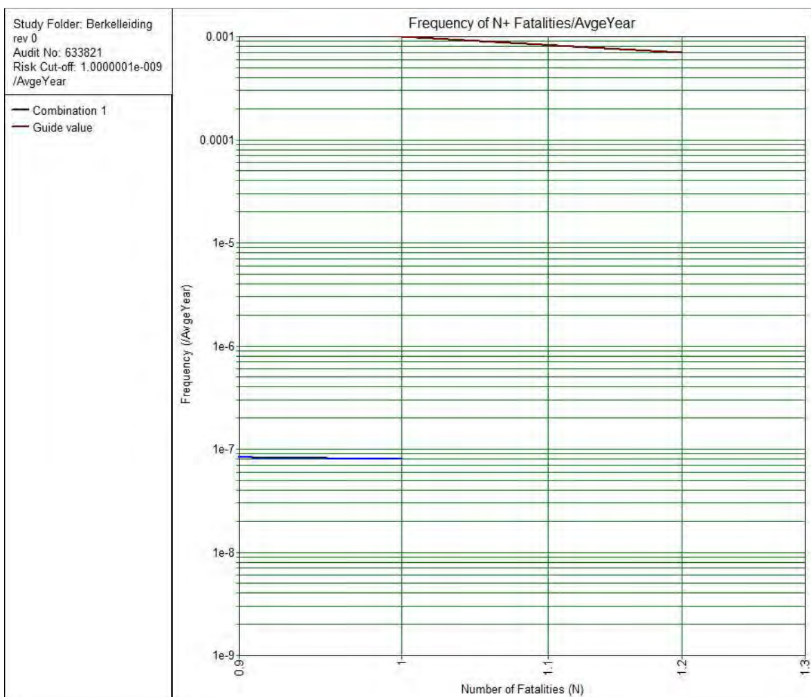
Figuur 4.6: Groepsrisico bij locatie Berkel
