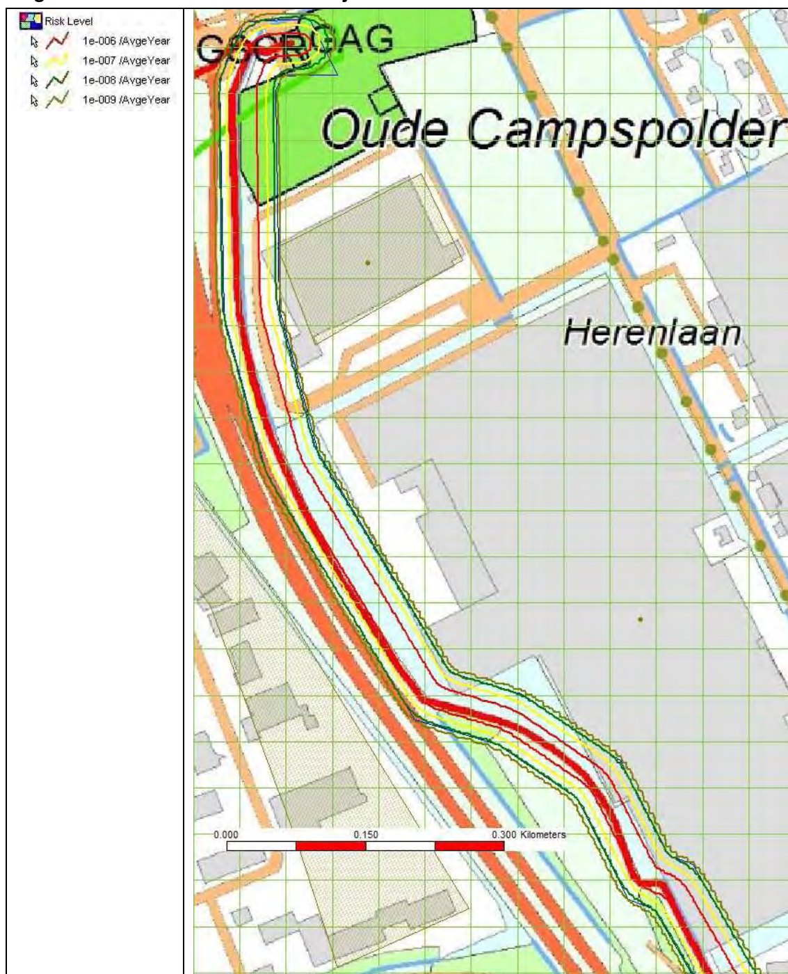
Figuur 4.3: Risico Contouren nabij A20.
