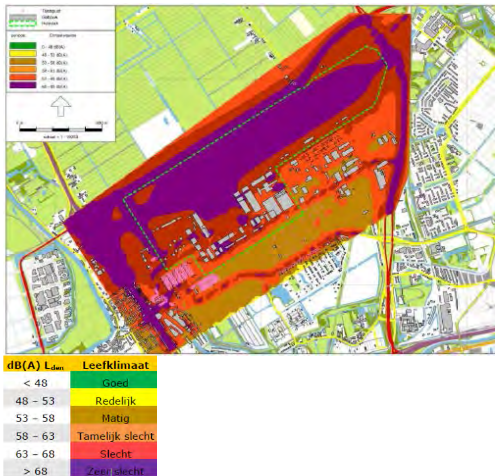
Figuur 5.10 Cumulatieve L den -contouren behorende bij de planvariant 2024 (plangebied is met groene stippellijn aangegeven)
