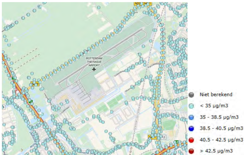
Figuur 6.3 Concentratie fijn stof ( PM_{10} ) in 2015 en 2020 (bron: www.nsl-monitoring.nl , plangebied donkerder weergegeven)
