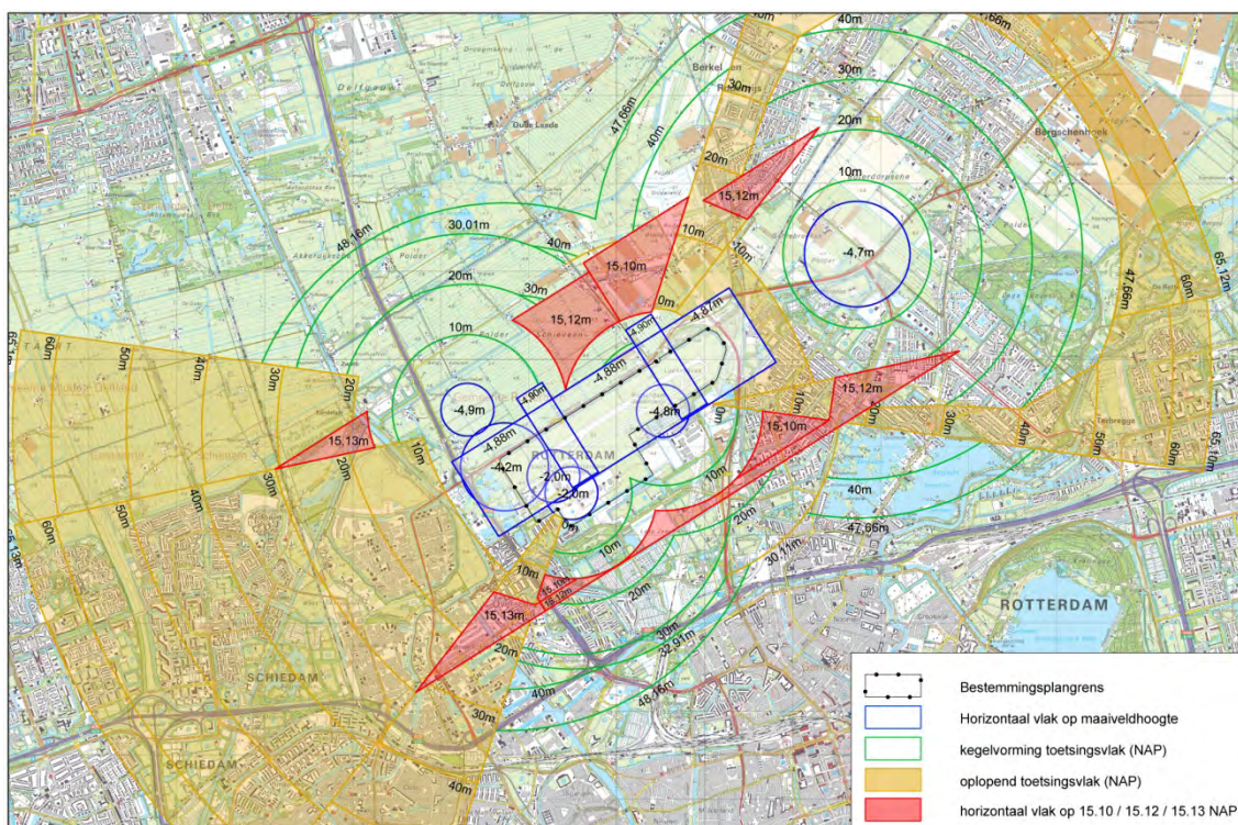
Figuur 9.2 Toetsingsvlakken van navigatie en communicatieapparatuur
