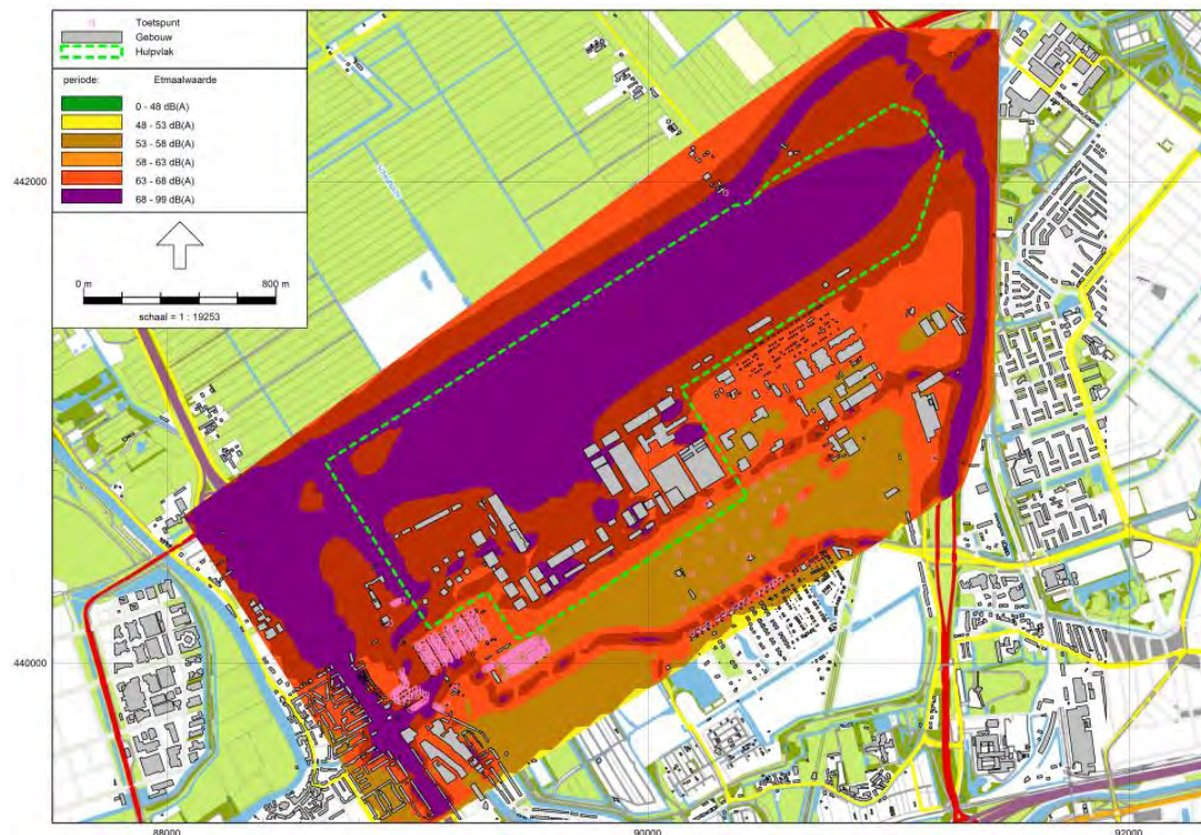
Figuur 20 Cumulatieve L_{den} -contouren behorende bij de planvariant 2024 (plangebied is met groene stippellijn aangegeven).
