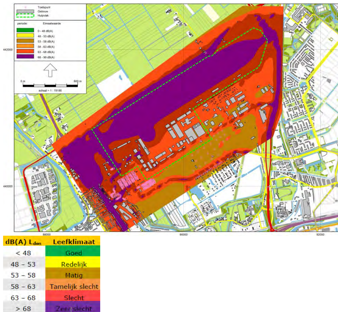
Figuur 5.6 Cumulatieve L_{den} -contouren in de autonome situatie (plangebied is met groene stippellijn aangegeven)
