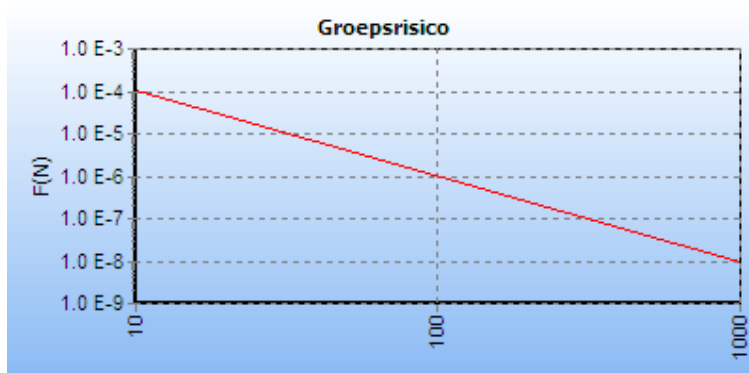
5.2 Figuur 5.4 FN curve voor W-530-01 van N.V. Nederlandse Gasunie voor de kilometer tussen stationing 2370.00 en stationing 3370.00
