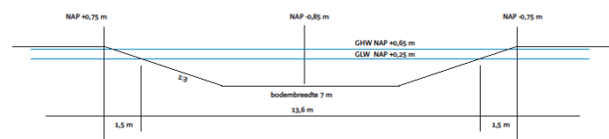
PROFIEL 10: nieuwe geul bij kruising middenrug
