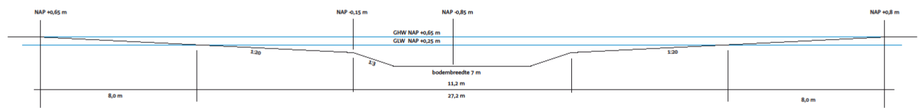
PROFIEL 5: nieuwe geul ter hoogte van noordelijk gelegen diep watervlak
