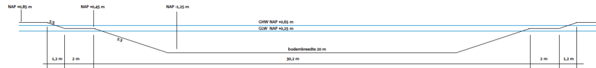
PROFIEL 1: nieuwe geul buitendijks
