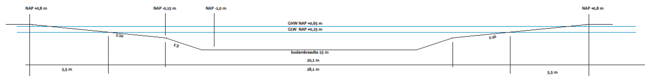
PROFIEL 3: nieuwe geul ter hoogte van voormalige kreekrug
