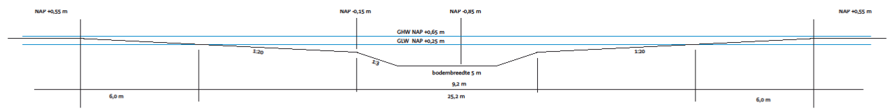
PROFIEL 6 en 7: nieuwe geul ter hoogte van zuidelijk gelegen diep watervlak
