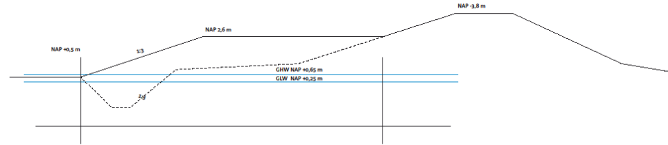
PROFIEL 12: aanberming westzijde hoofdwaterkering
