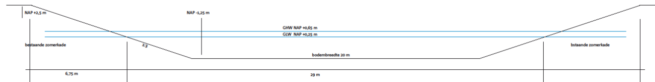
PROFIEL 2: nieuwe geul ter hoogte doorsnijding bestaande zomerkade
