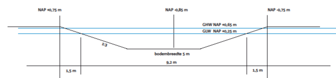
PROFIEL 8 en 9: nieuwe geul bij kruising middenrug
