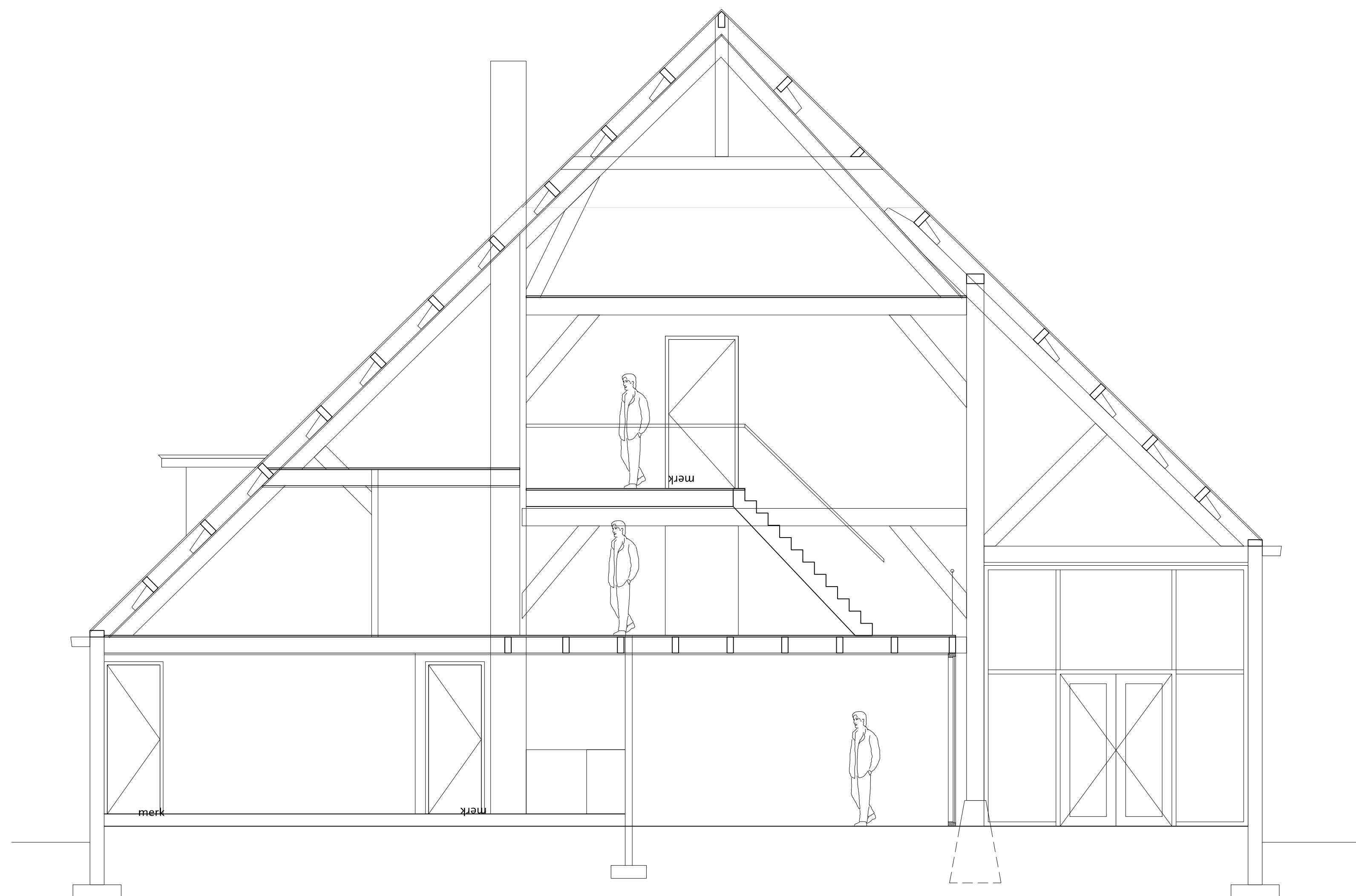
Doorsnede C-C
