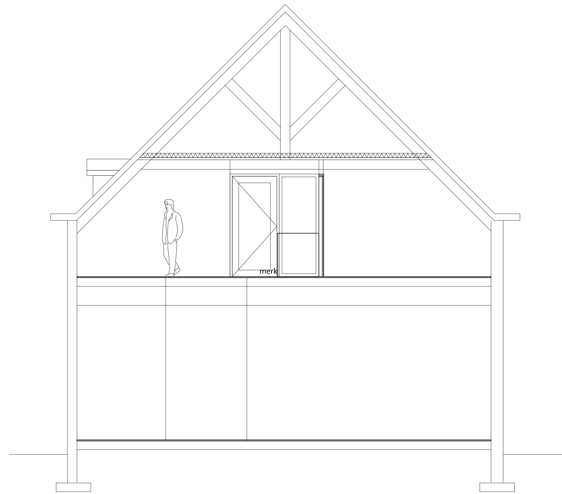
Doorsnede E-E
