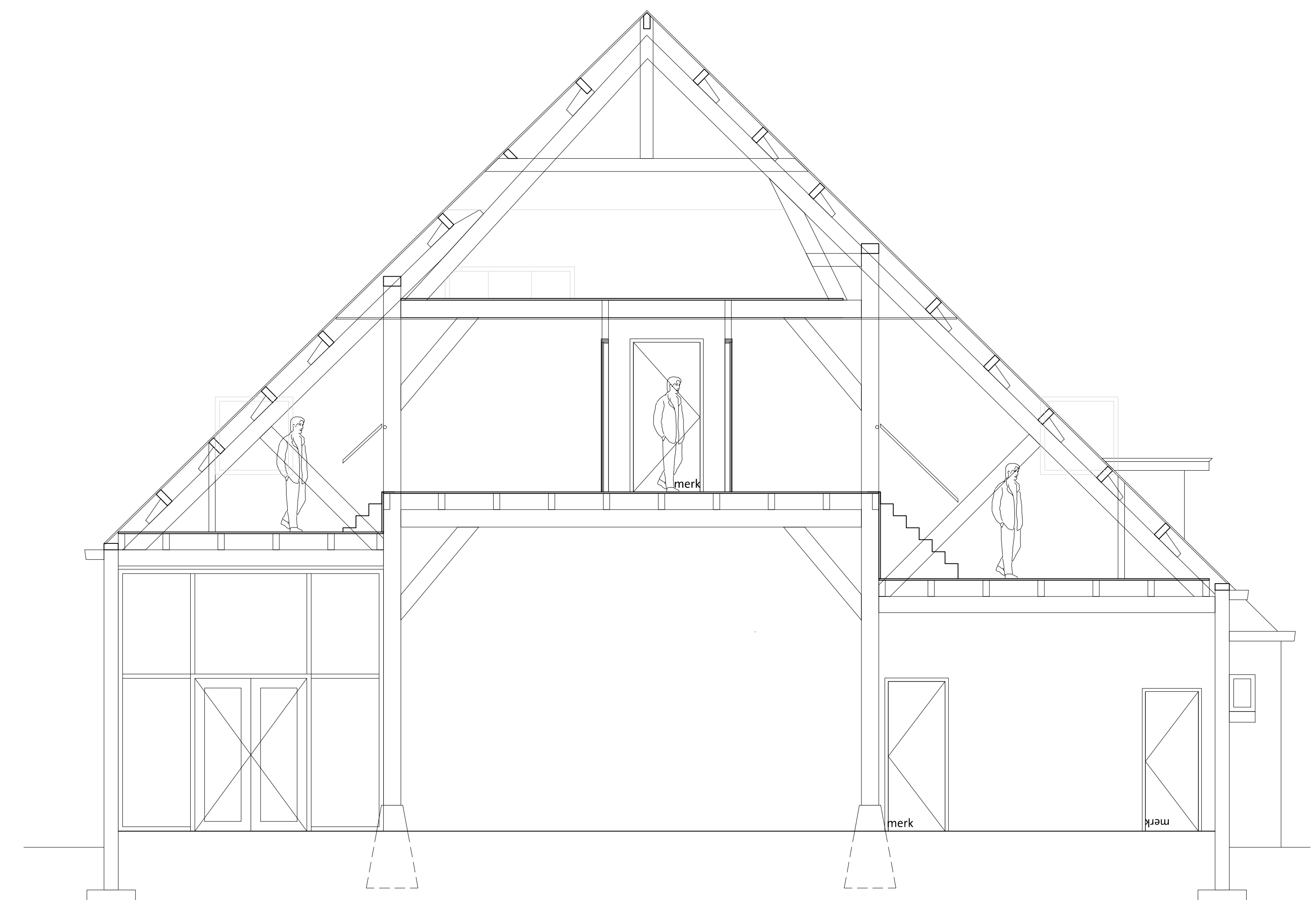
Doorsnede B-B
