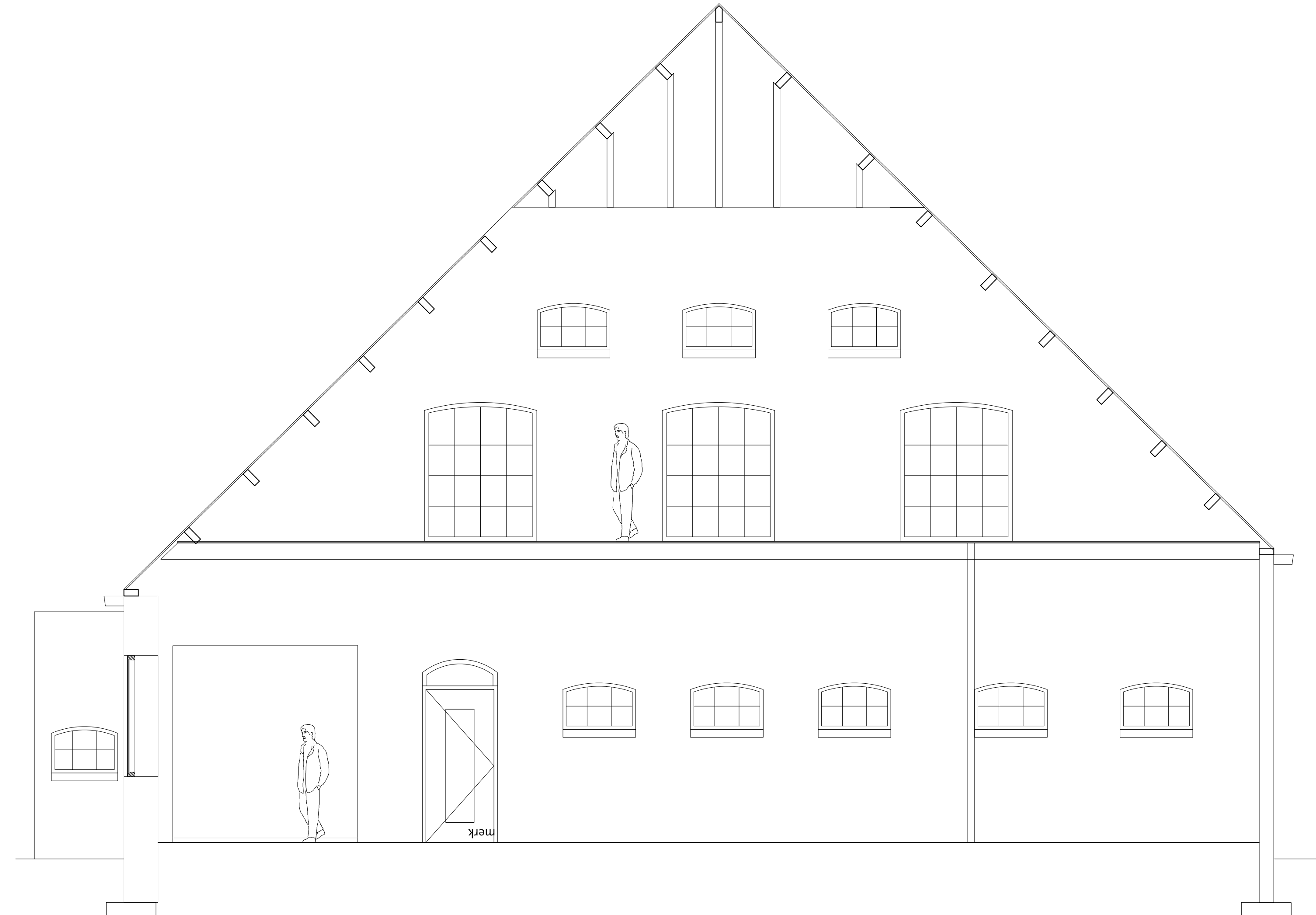
Doorsnede D-D
