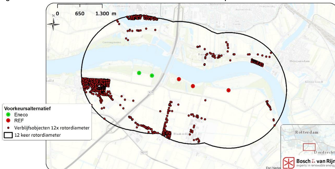
Figuur 9 Windturbinelocaties van het voorkeursalternatief voor windpark Oude Maas
