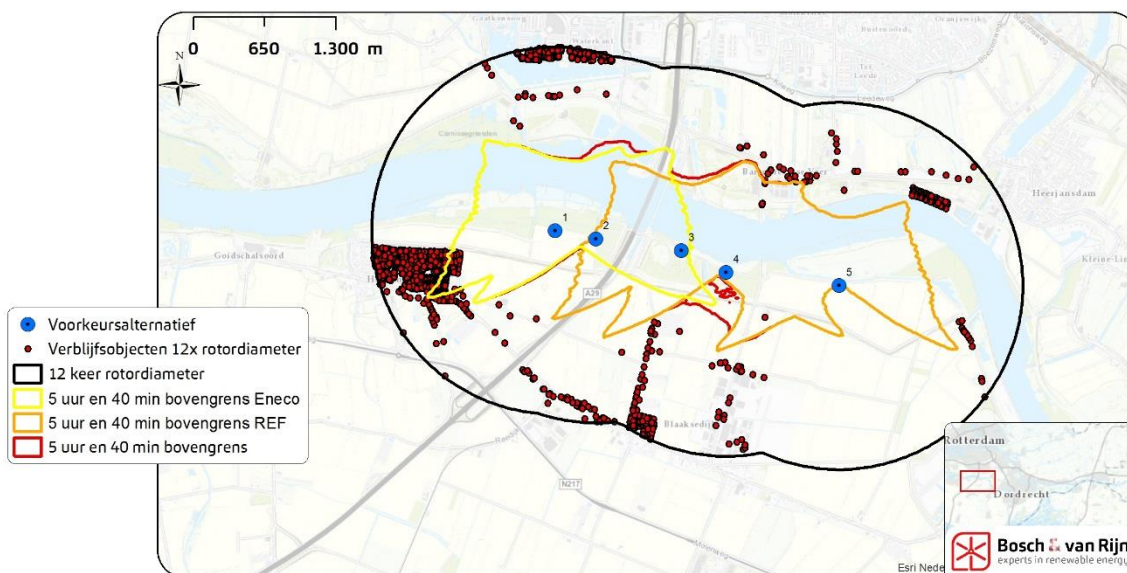
Figuur 11 5 uur en 40 minuten slagschaduwcontour van beide inrichtingen voor de bovengrens
