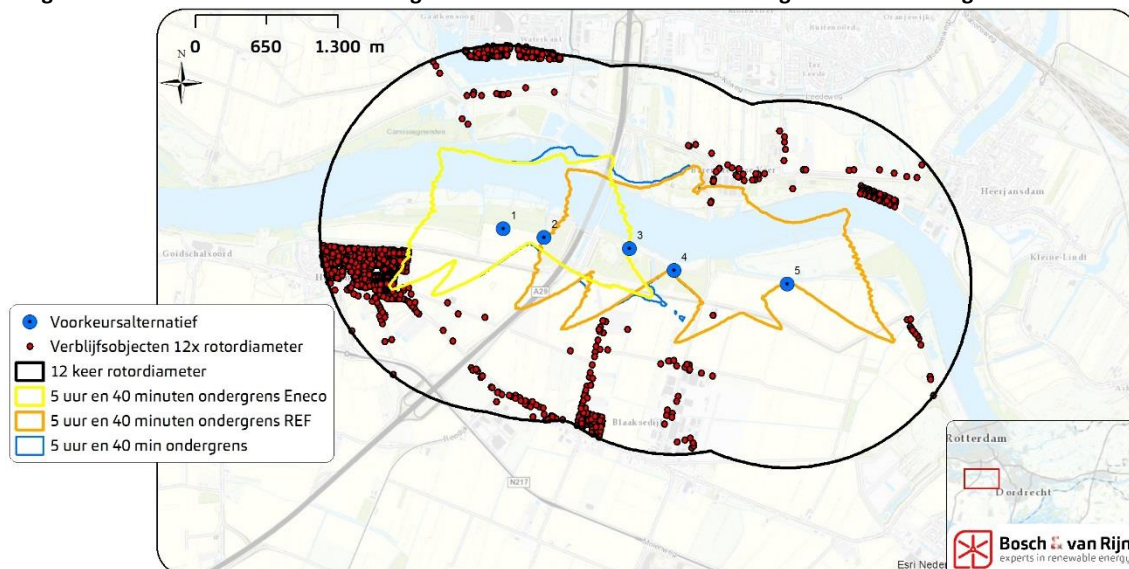
Figuur 12 5 uur en 40 minuten slagschaduwcontour van beide inrichtingen voor de ondergrens
