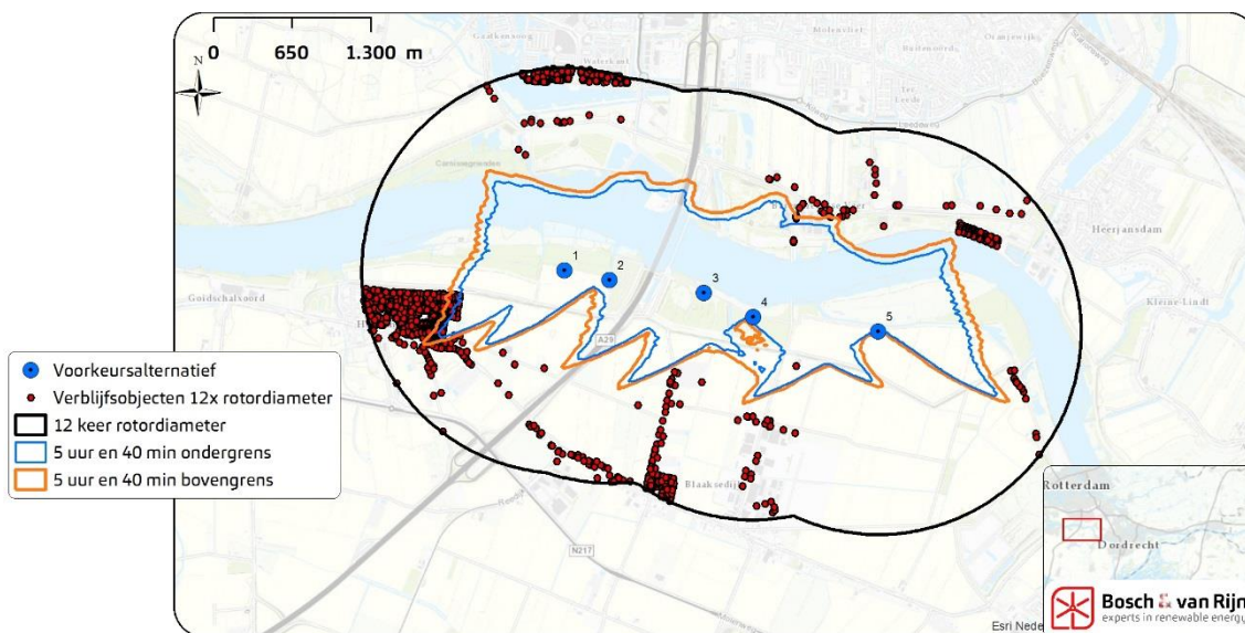
Figuur 10 5 uur en 40 minuten slagschaduwcontour van onder- en bovengrens
