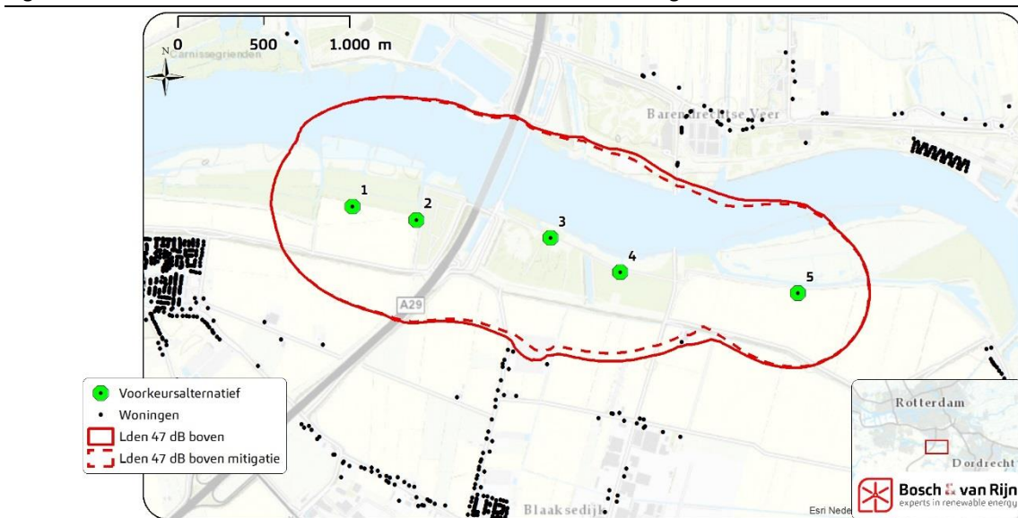
Figuur 9 Geluidscontour Lden 47 dB. Met en zonder reductiemaatregel NRO 104 in de nacht.
