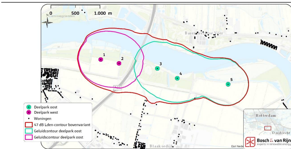
Figuur 10 Geluidscontouren van de twee deelparken: 2 windturbines ten westen van de snelweg en 3 windturbines ten oosten ervan.
