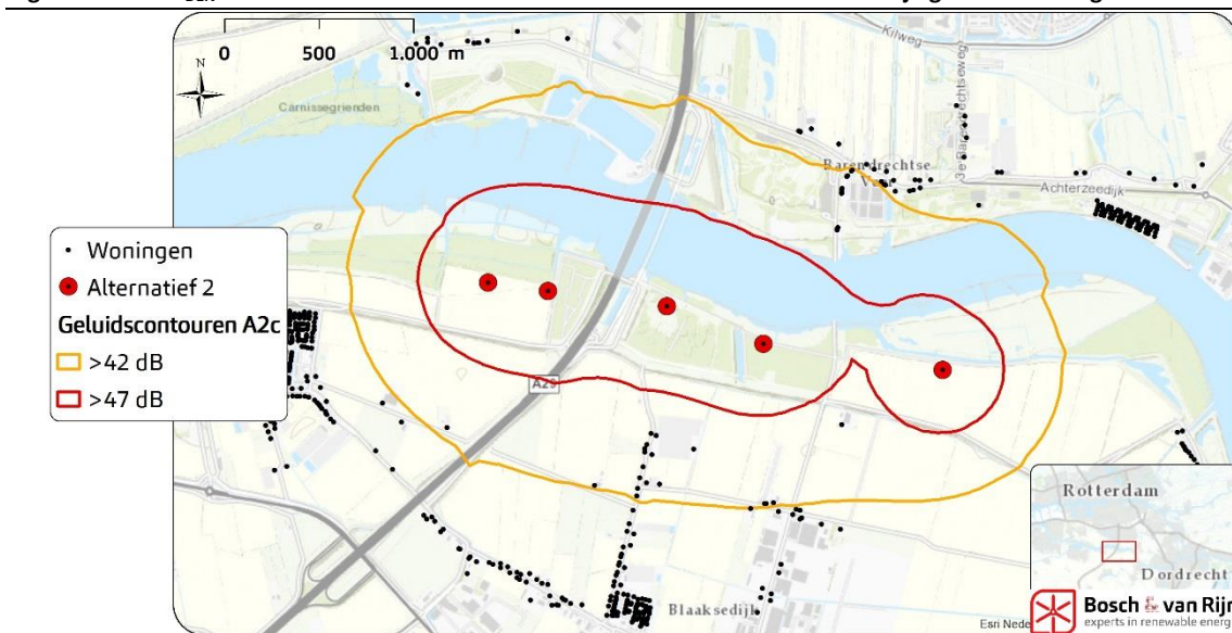
Figuur 6 L_{DEN} 47 en 42 dB-contour van de Alternatief A2c ter illustratie. Zie Bijlage C voor overige contouren.
