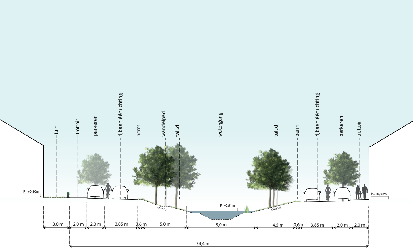
Profiel 8
