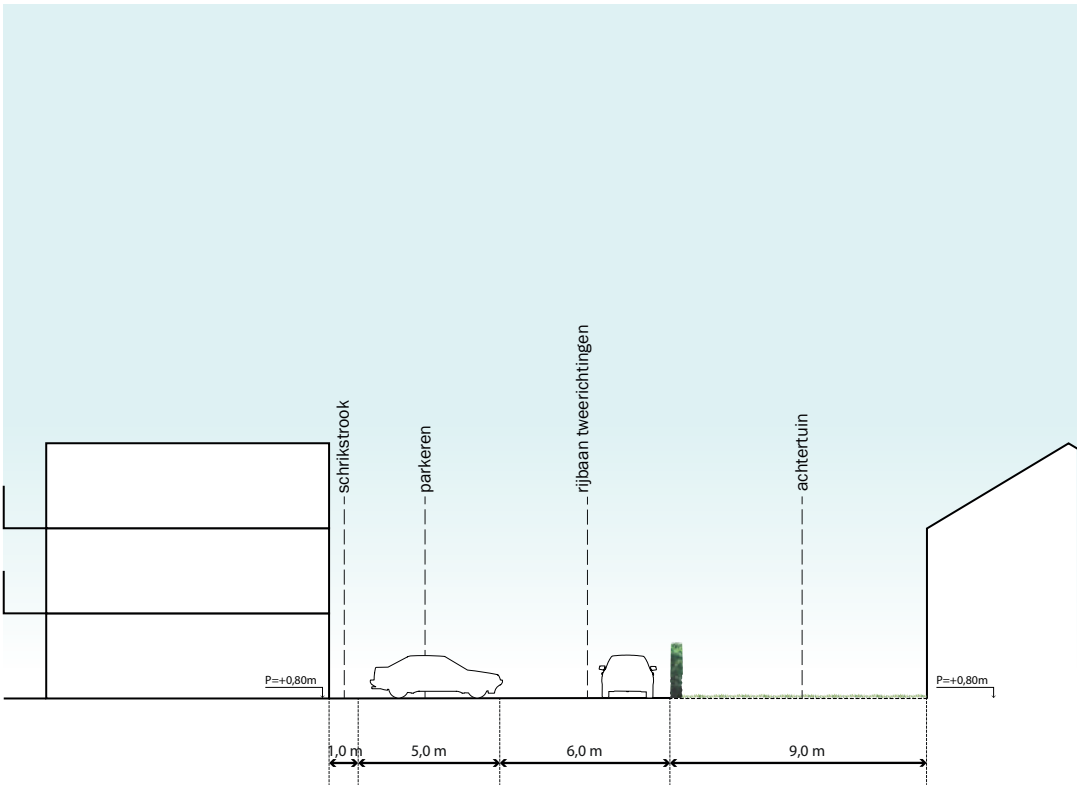
Profiel 6
