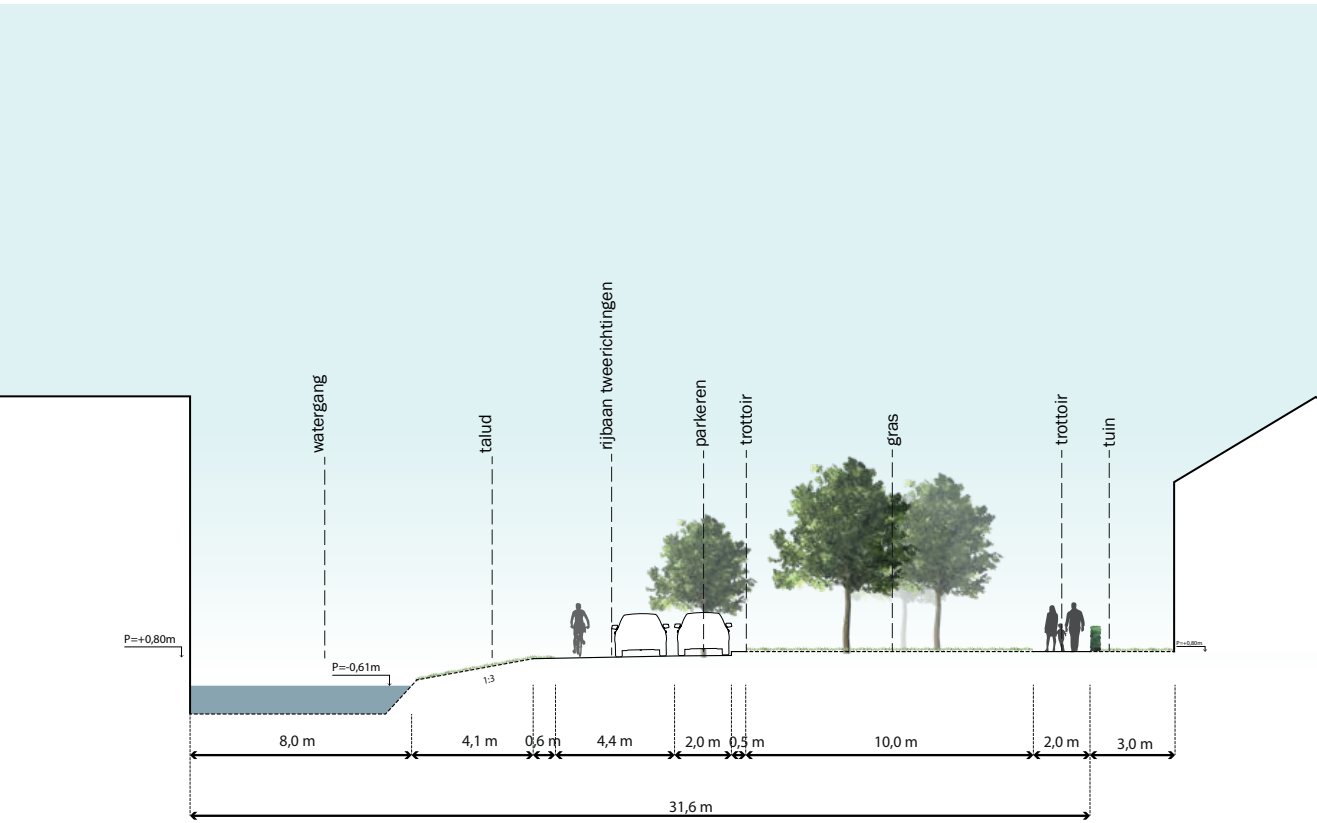
Profiel 7
