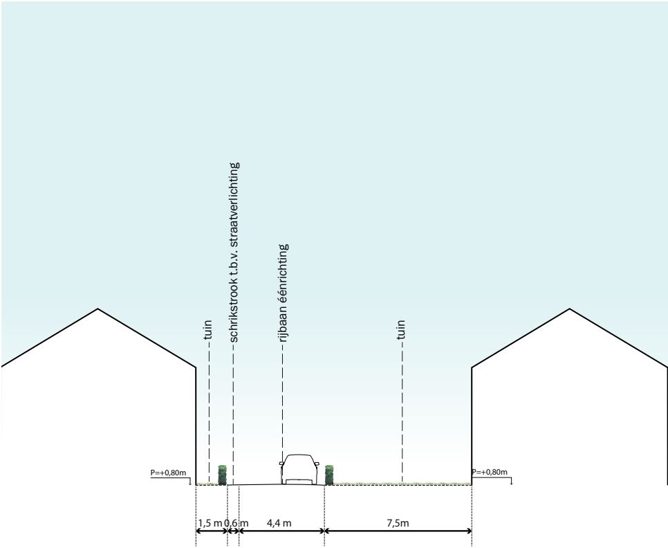
Profiel 2
