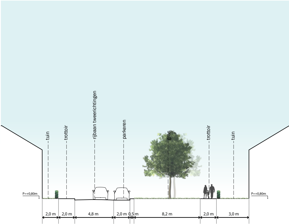
Profiel 10
