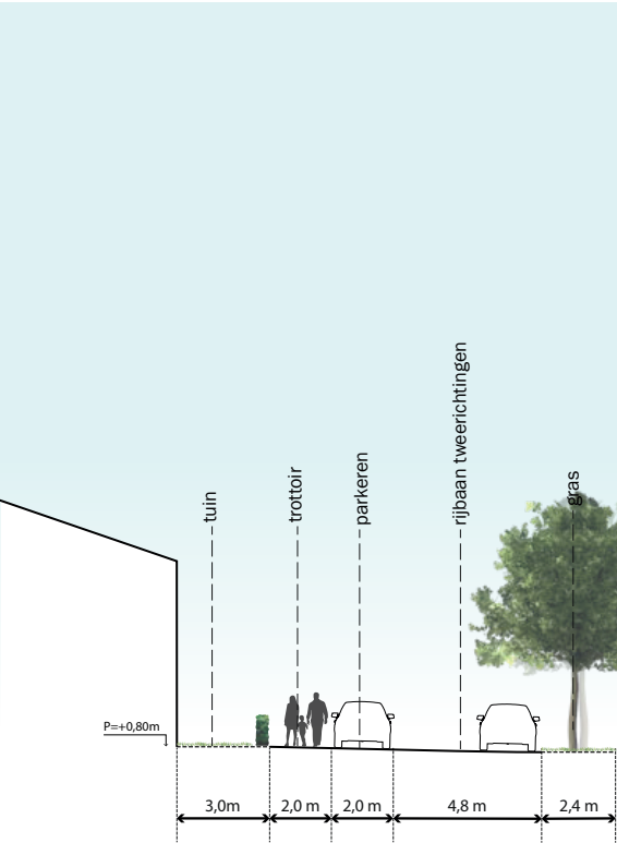
Profiel 9
