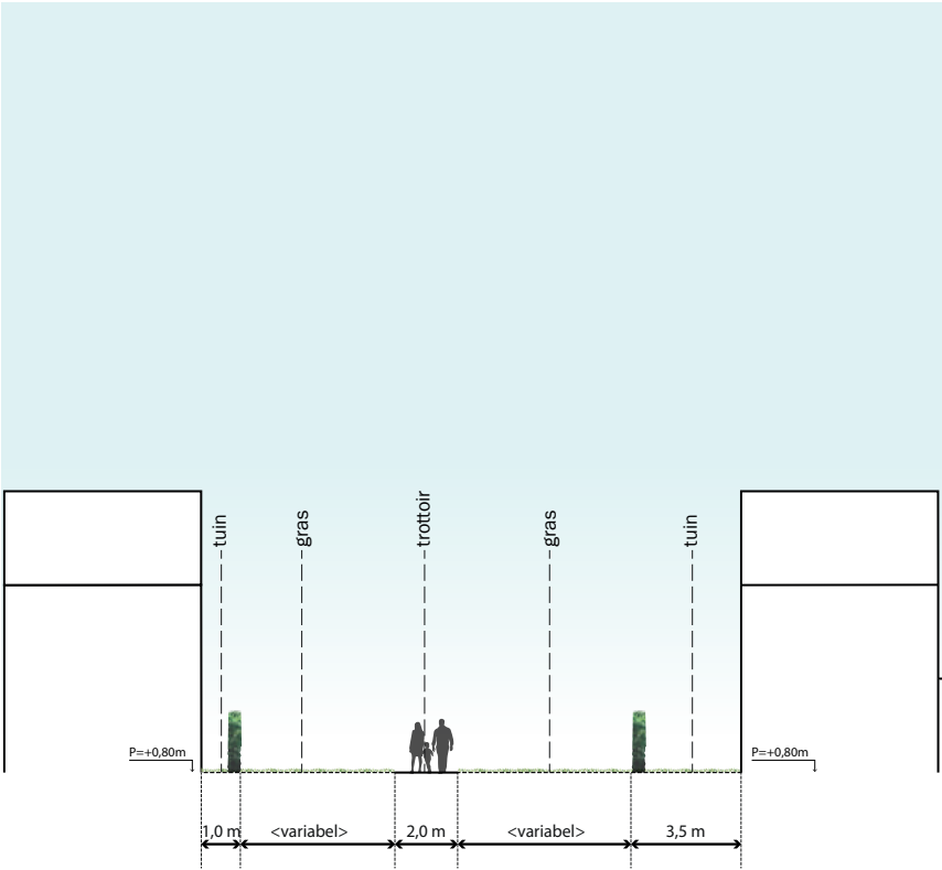
Profiel 4
