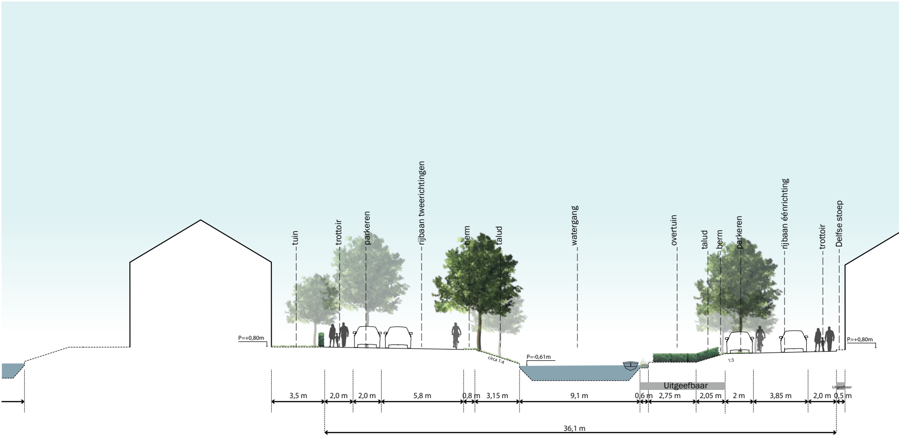
Profiel 1
