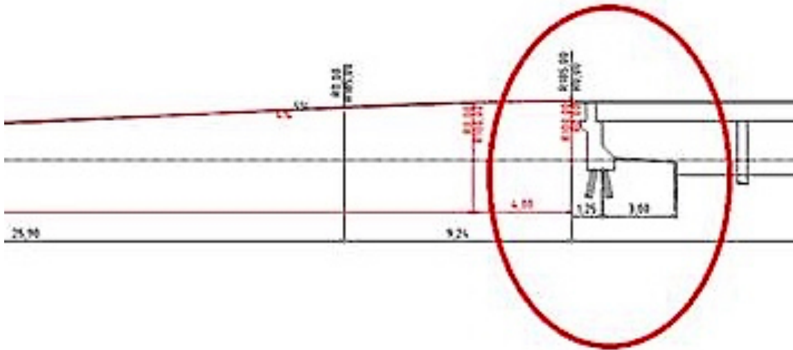
figuur 4 detailtekening van de ruimte onder de brug langs de Haarlemmertrekvaart. De droge strook onder de brug is 3 m breed en de hoogte bedraagt ca 1 m.
