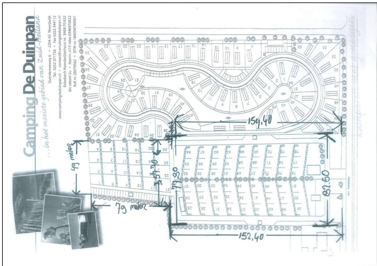
Figuur 2. Plansituatie.
