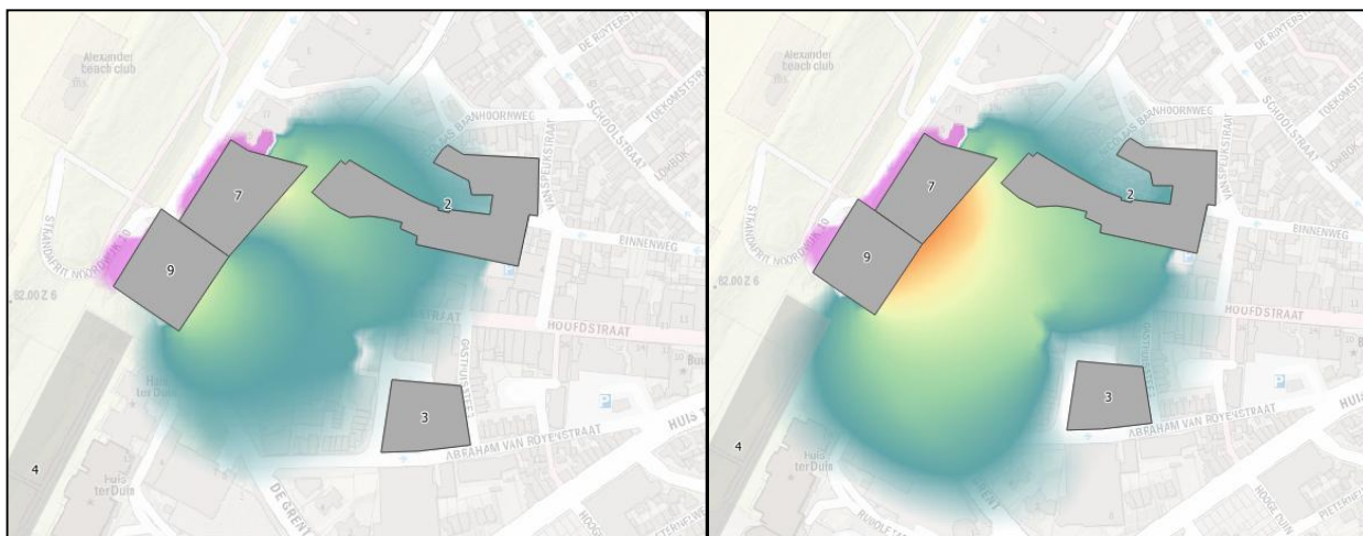
Figuur 2: voorbeeldweergave effect combinatie kelders. In de linker figuur zijn de onderlinge effecten van de kelders 2,3,7 en 9 weergegeven. In de rechter figuur de effecten bij de gecombineerde aanwezigheid van de kelders.
