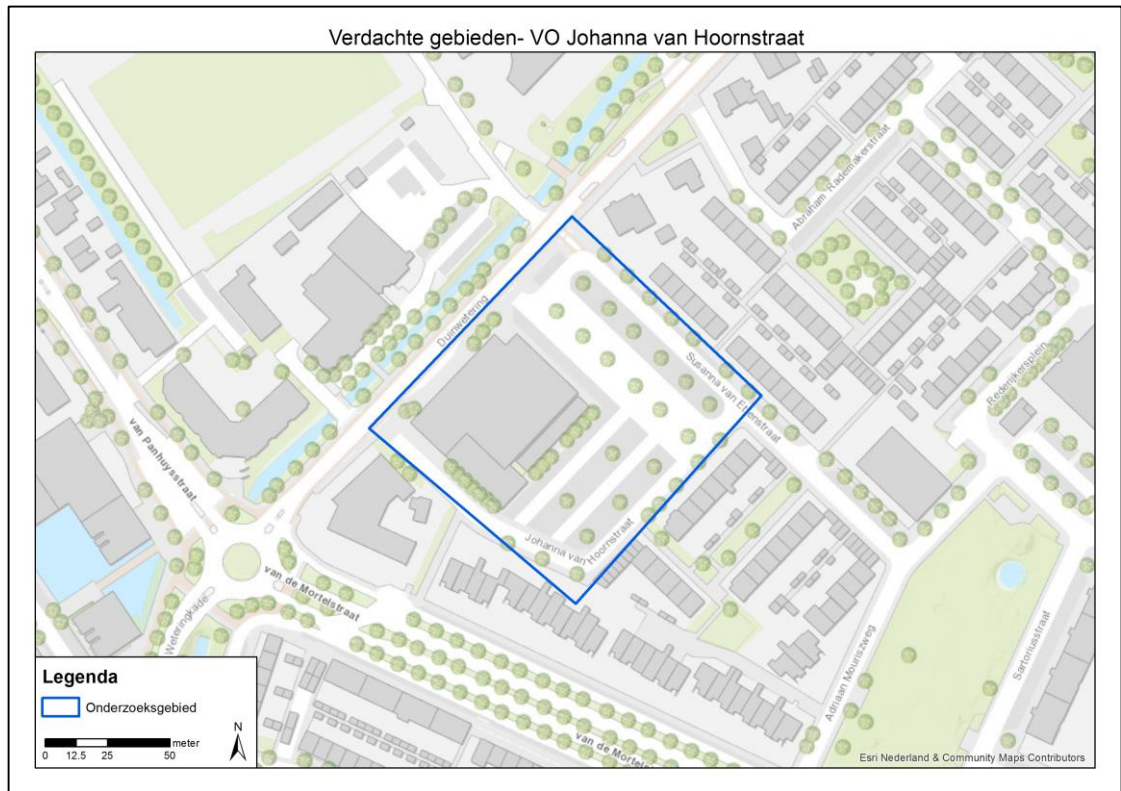
Afbeelding 2: CE bodembelastingkaart Johanna van Hoornstraat Noordwijk.
