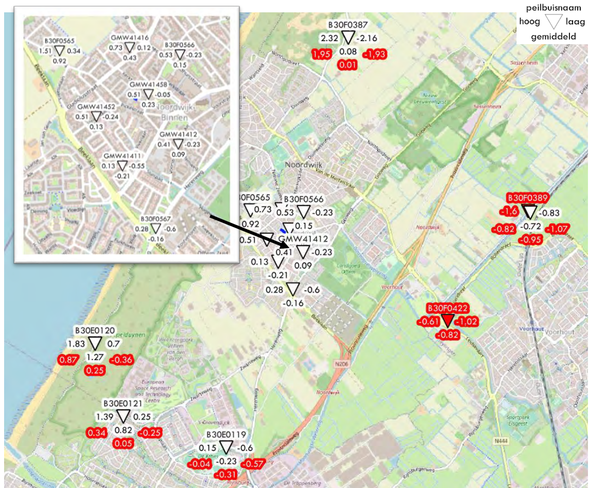
figuur 6 - grondwaterstand t.o.v. NAP per geanalyseerde peilbuis (wit = freatisch/watervoerende laag 1, rood = watervoerende laag 2)
